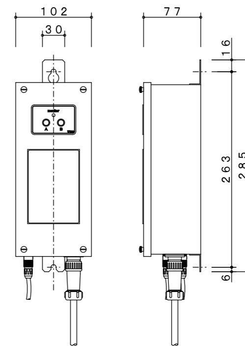
太陽電池制御部詳細図 S = 1 / 5
