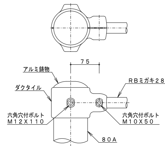
A詳細図 S=1/5
