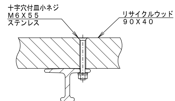
A-A断面図 S=1/3
