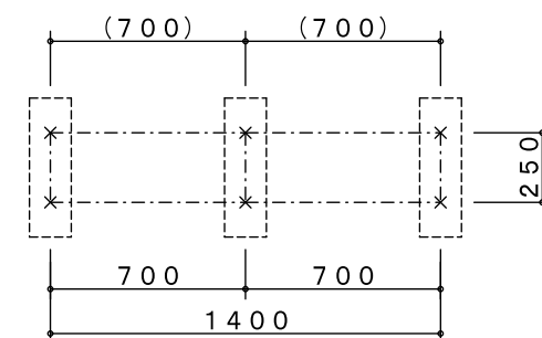
アンカー位置参考図 S=1/30
