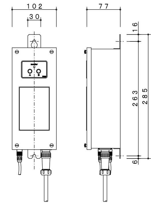
太陽電池制御部詳細図 S = 1 / 5
