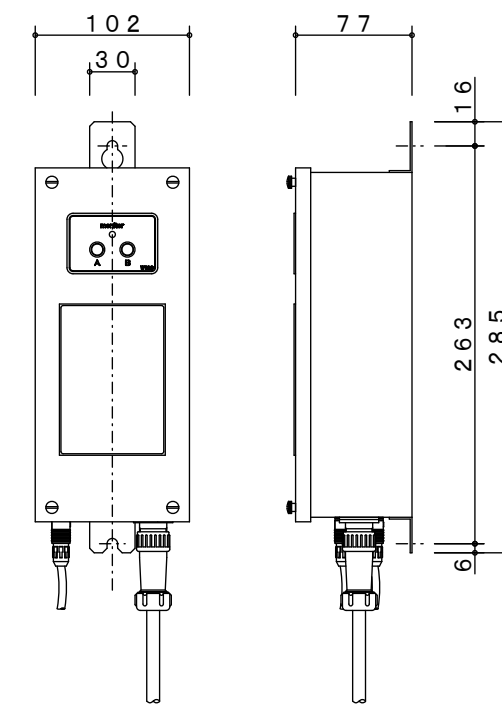
太陽電池制御部詳細図 S = 1 / 5
