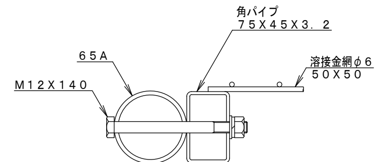
B詳細図 S=1/4
