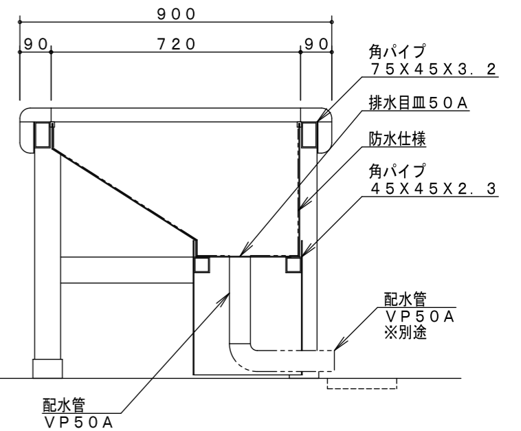
A-A' 断面図
