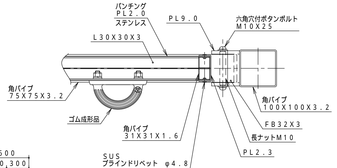
ボード部 断面詳細図 S = 1 / 6
