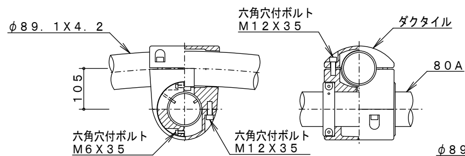
A詳細図 S=1/10
