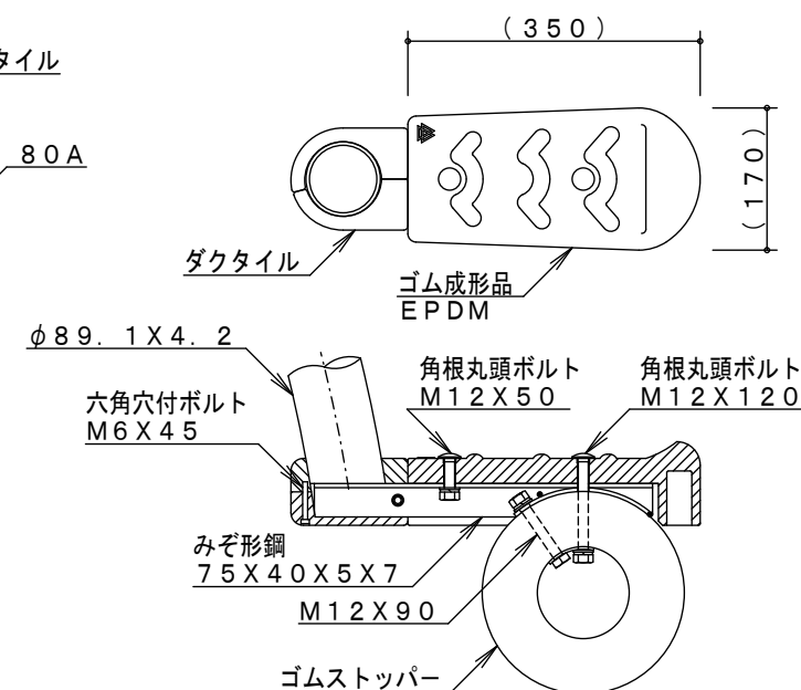
B詳細図 S=1/10
