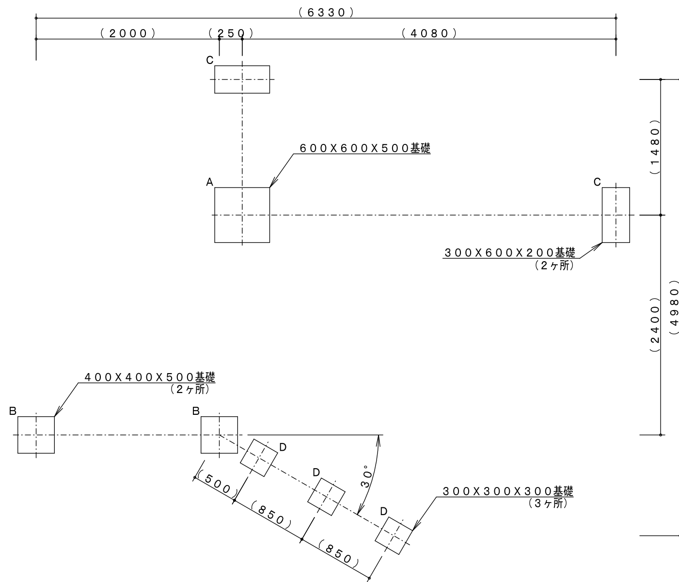
基礎平面図 S=1/40
