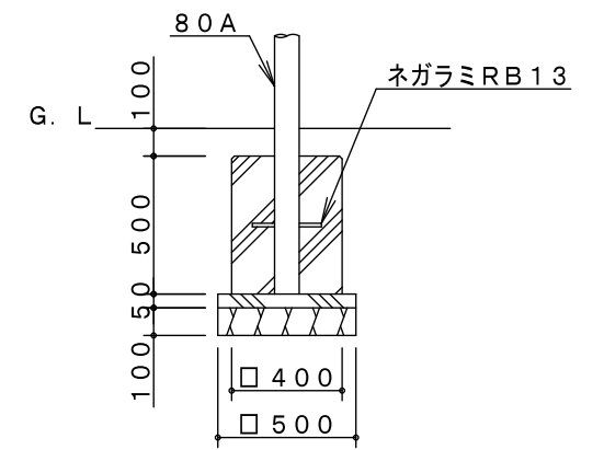
B基礎詳細図
