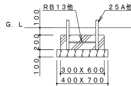
C基礎詳細図
