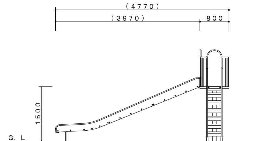
A-A' 矢視図
