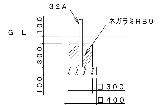
D基礎詳細図
