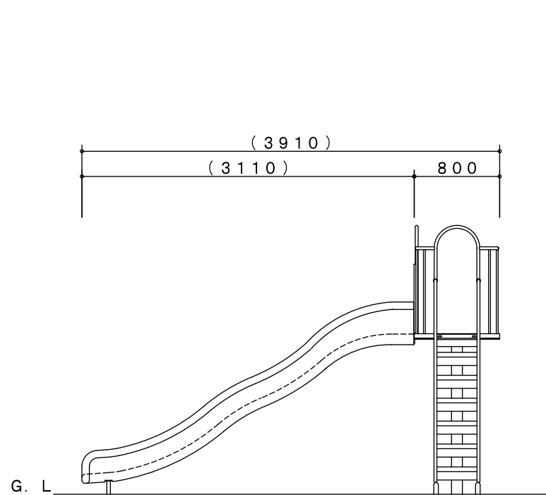
A-A' 矢視図
