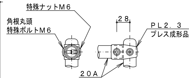
D詳細図 S=1/5
