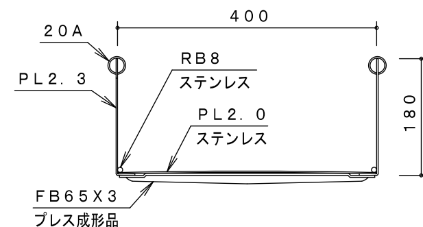
C断面図 S=1/8
