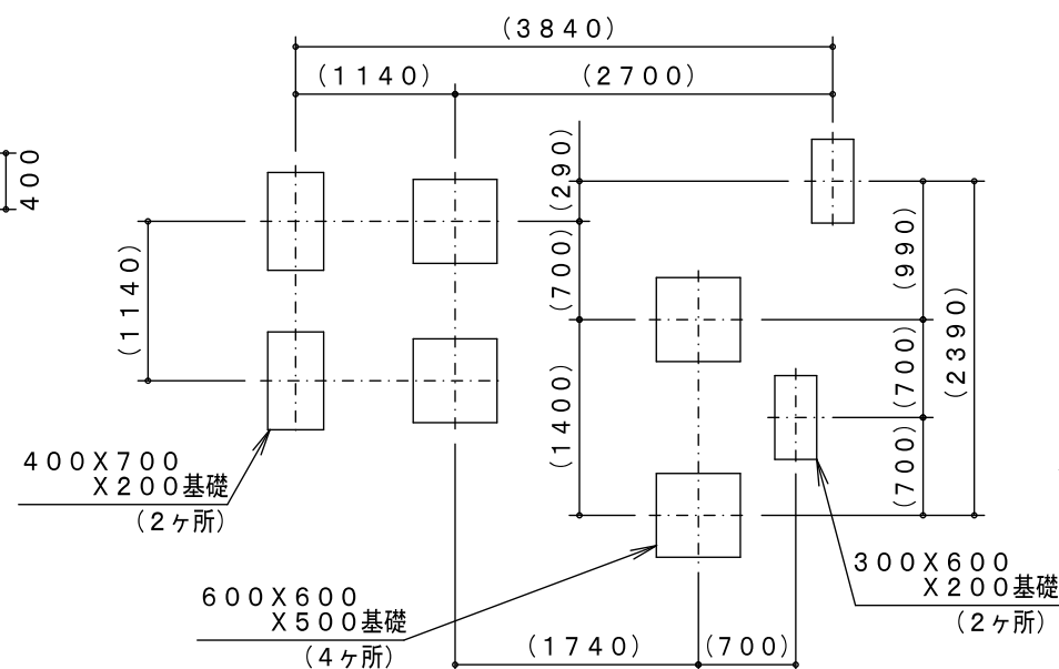
基礎平面図
