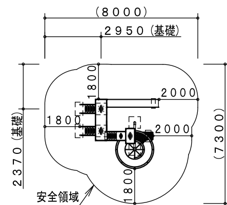
※製品外形からの寸法を示す 安全領域 S=1/200
