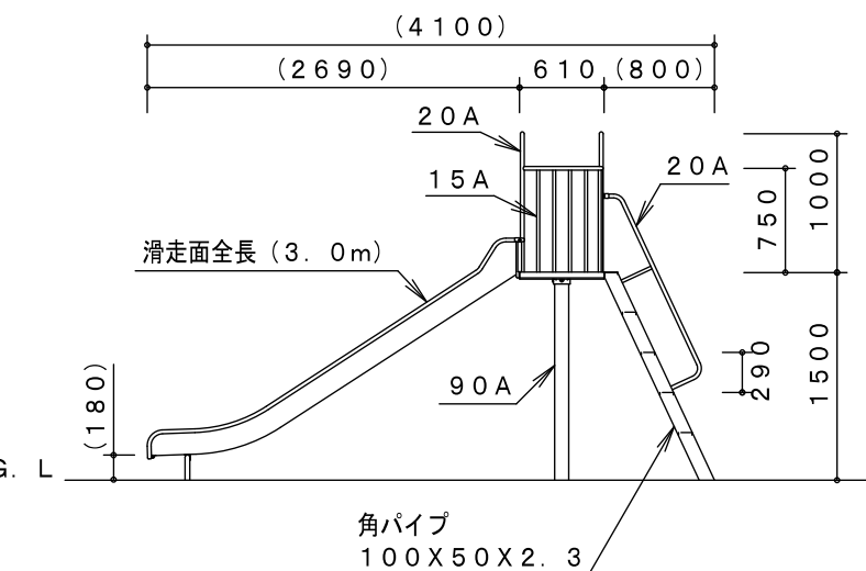
A矢視図
