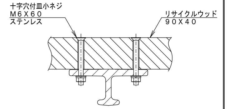
A-A断面図 S=1/3
