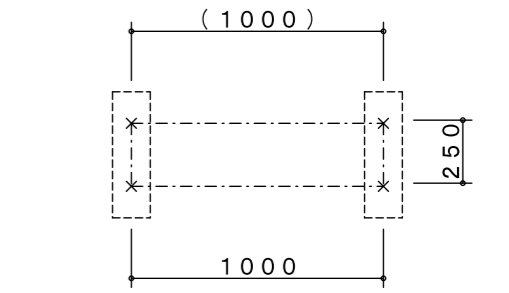
アンカー位置参考図 S=1/30
