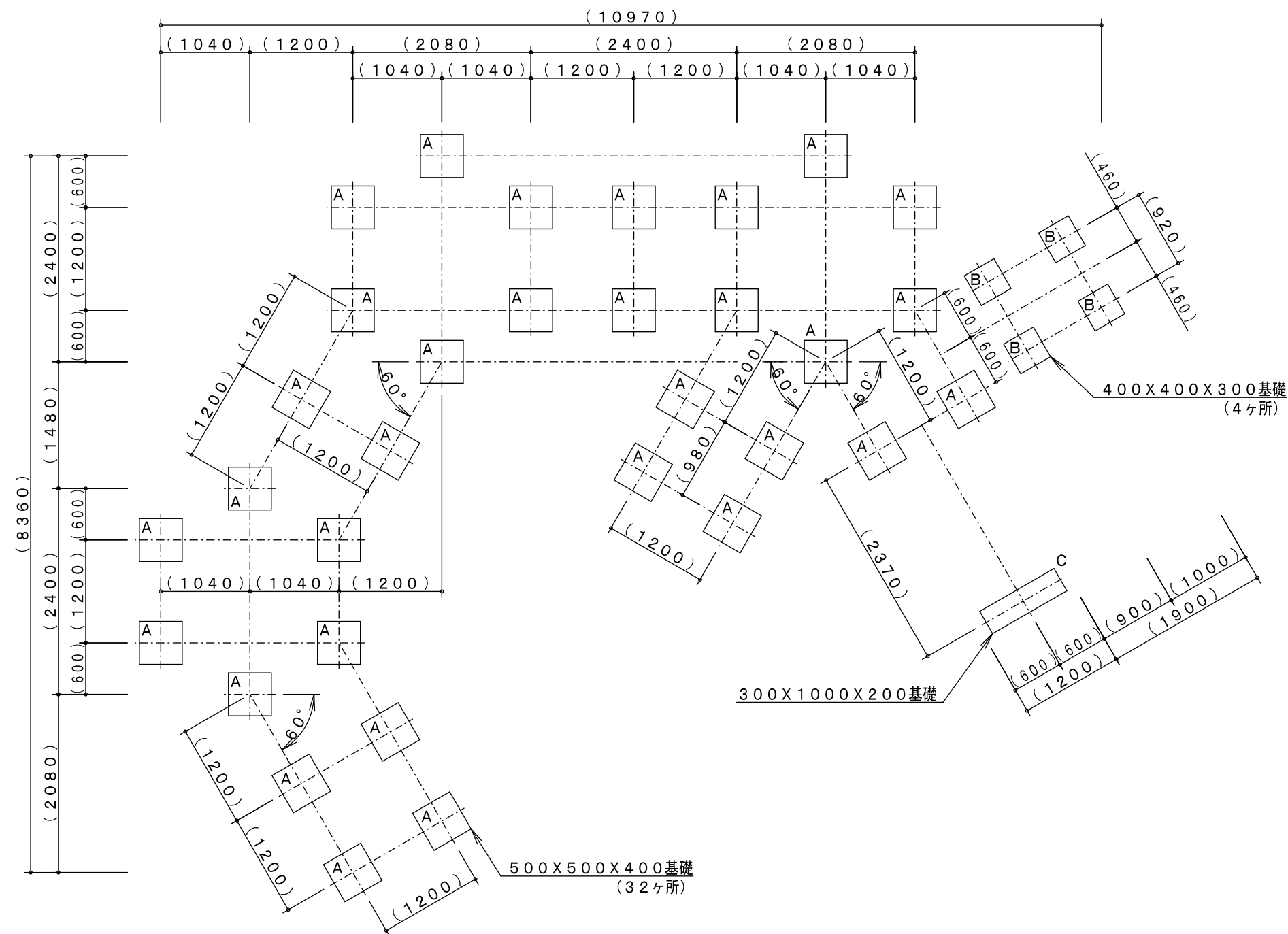
基礎平面図 S=1/60
