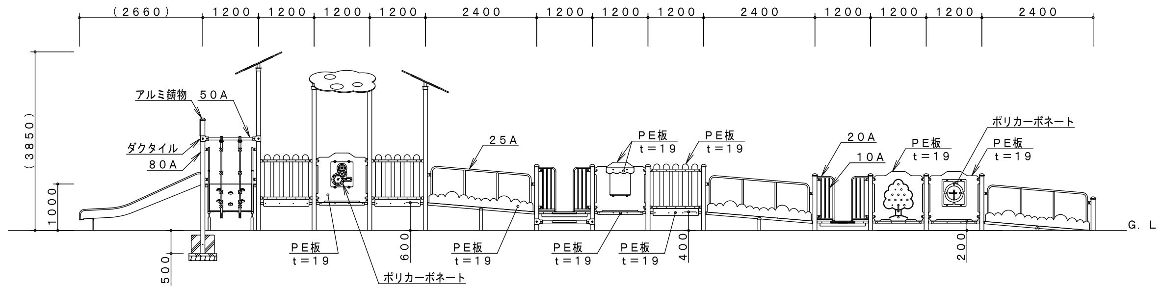
A-A' 展開図
