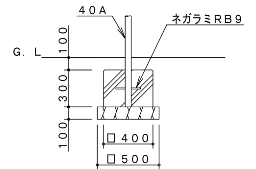
B基礎詳細図
