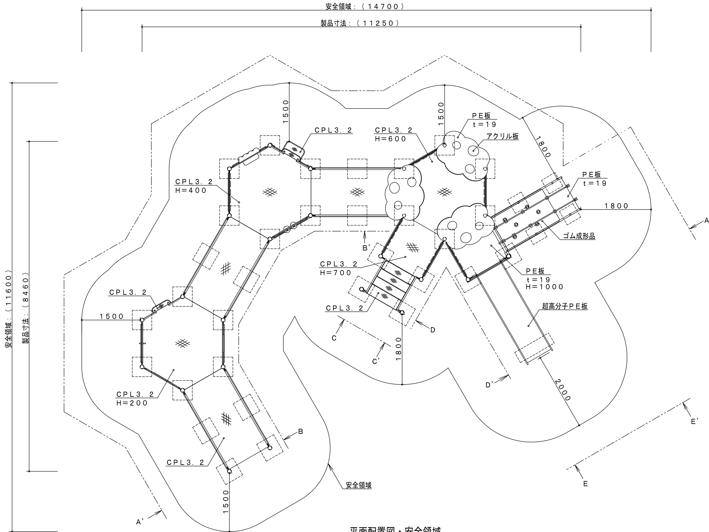
平面配置図・安全領域
