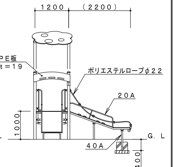
E-E' 矢視図
