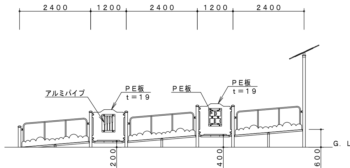
B-B' 展開図
