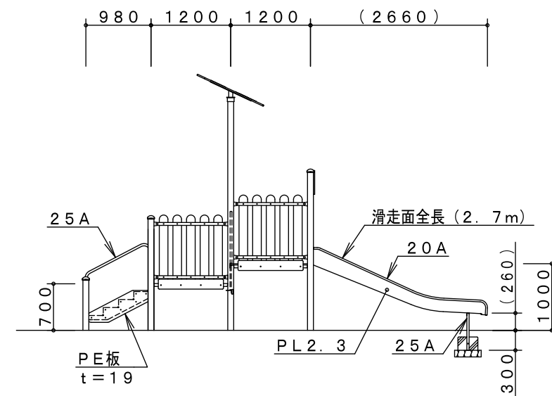
D-D' 展開図
