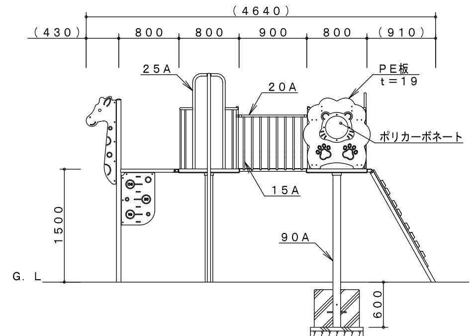
A-A' 矢視図
