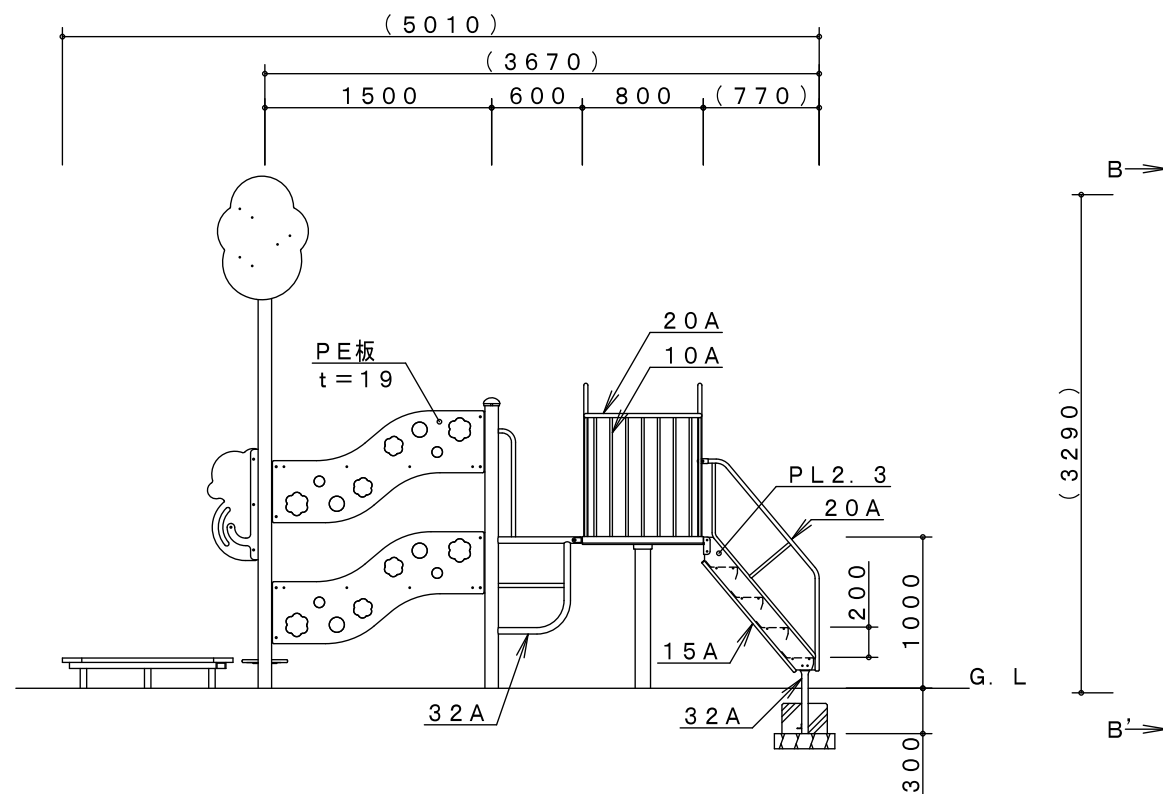
A-A' 矢視図
