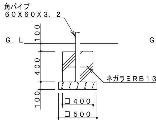
C 基礎詳細図
