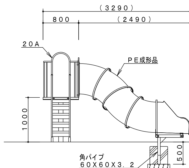
B-B' 矢視図
