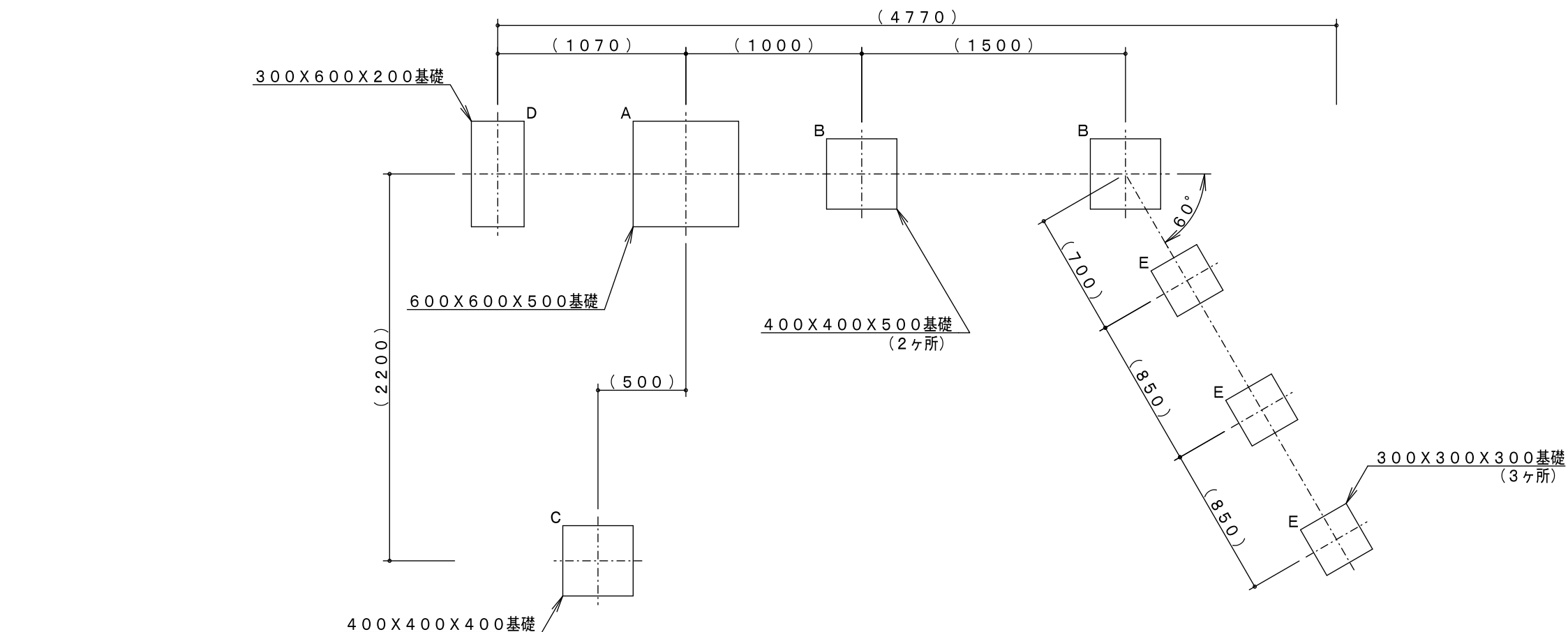
基礎平面図
