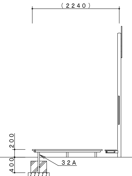
C-C' 矢視図
