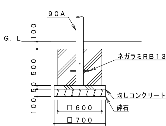
A 基礎詳細図
