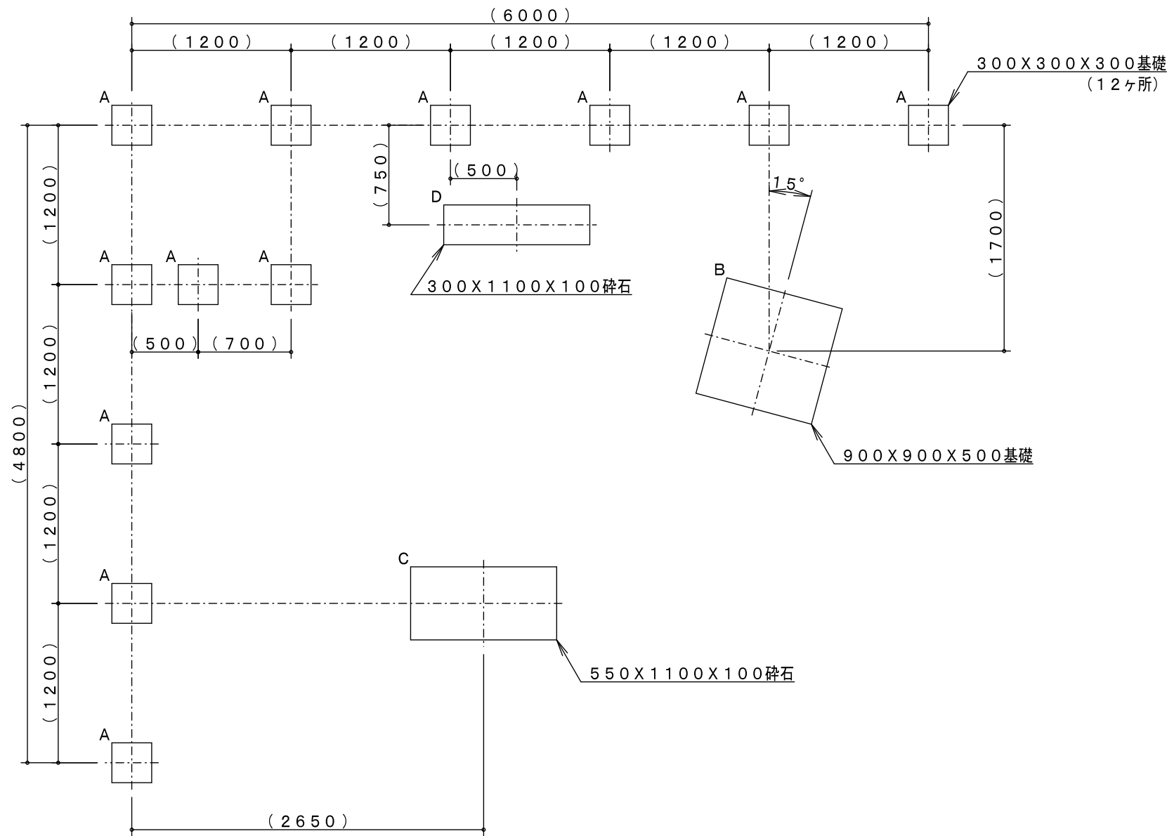
基礎平面図
