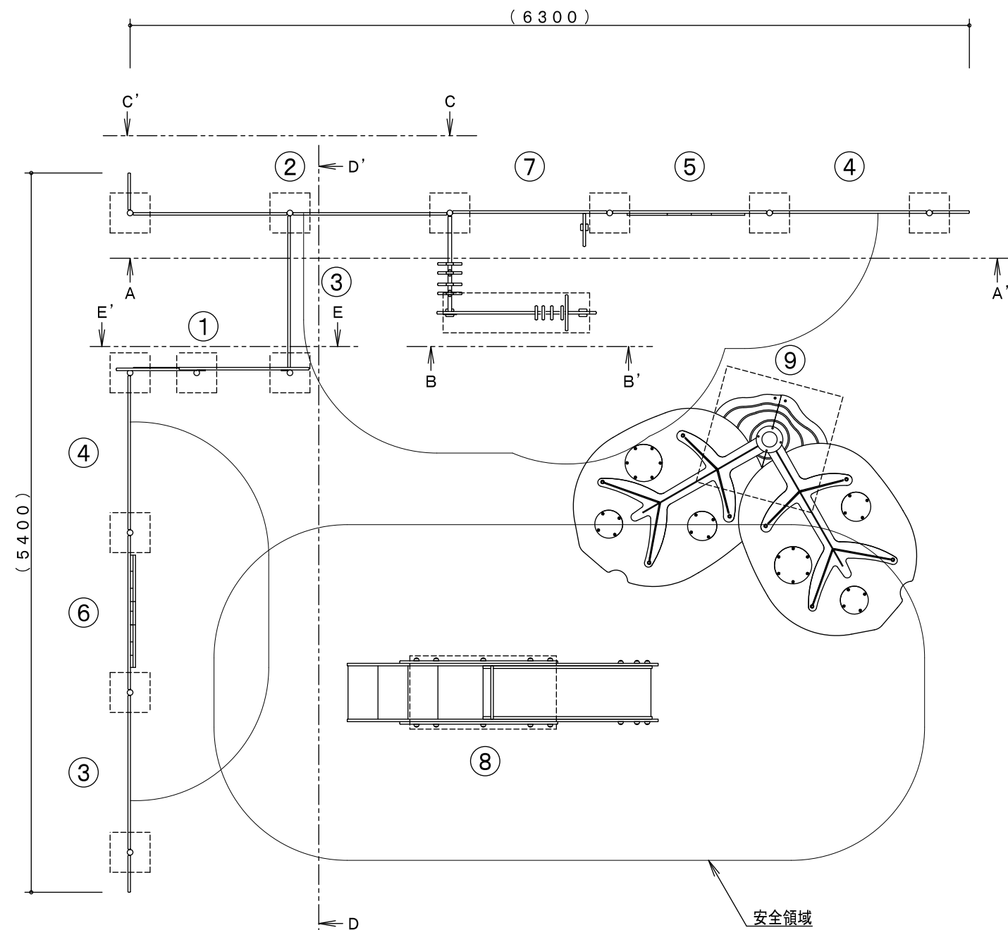
平面図
