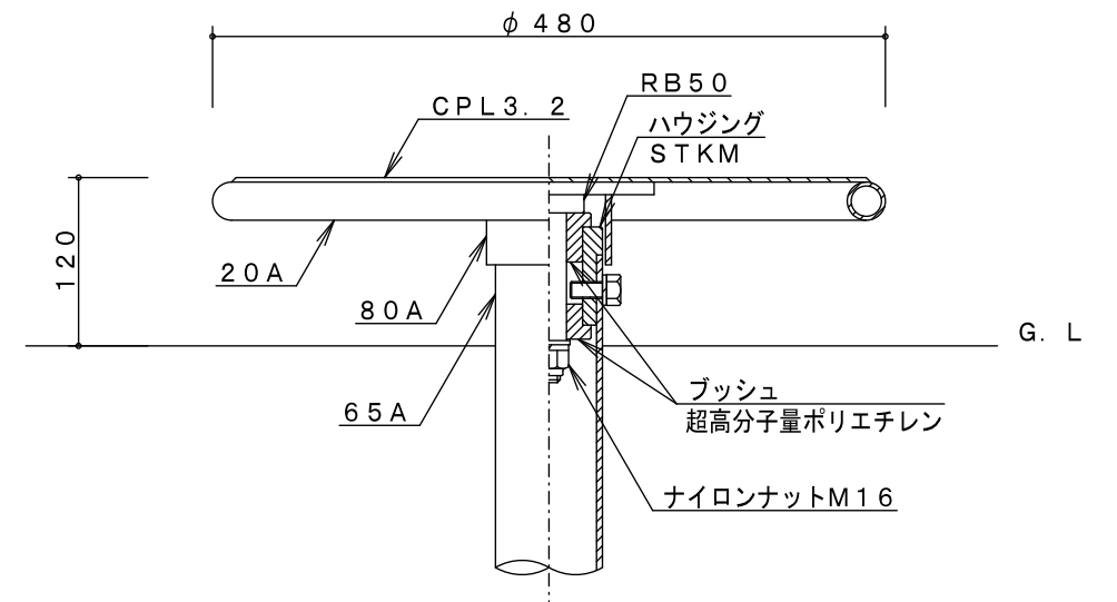
回転部詳細図 S = 1 / 6
