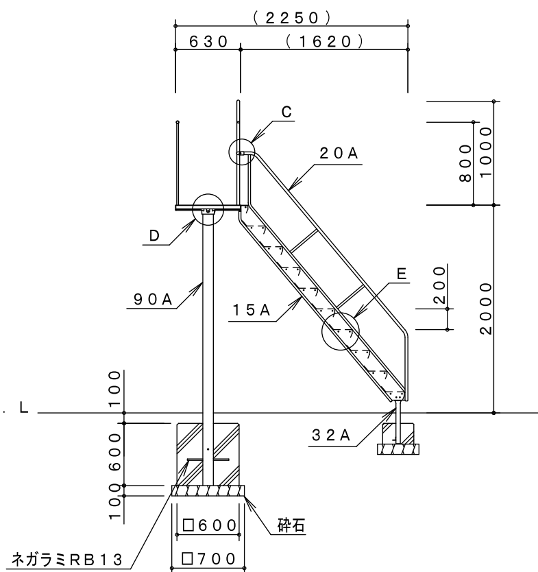
A矢視図
