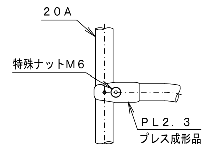
C詳細図 S=1/6
