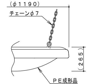
吊席 (C) 詳細図 S=1/20
