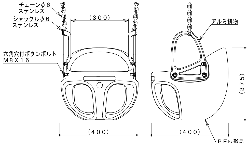
吊席 (A) 詳細図 S=1/10
