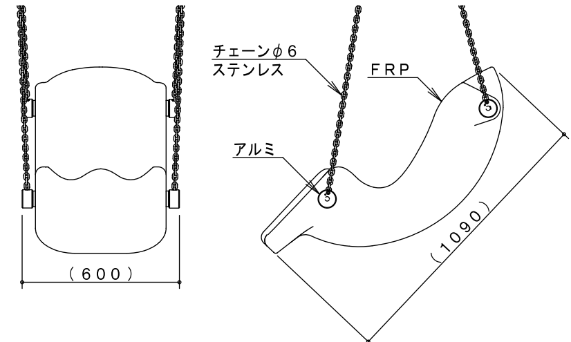
吊席 (B) 詳細図 S=1/20
