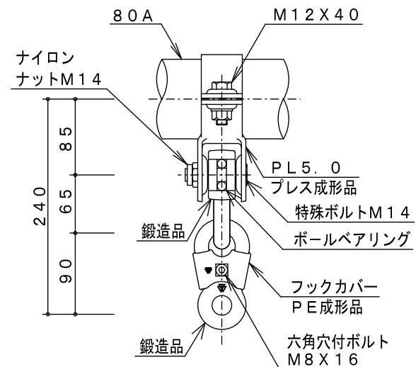
D詳細図 S=1/6
