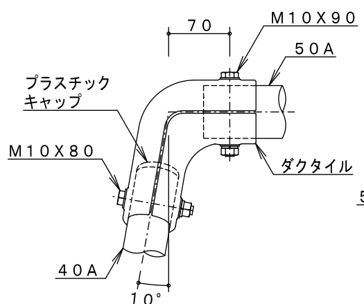
B詳細図 S=1/6
