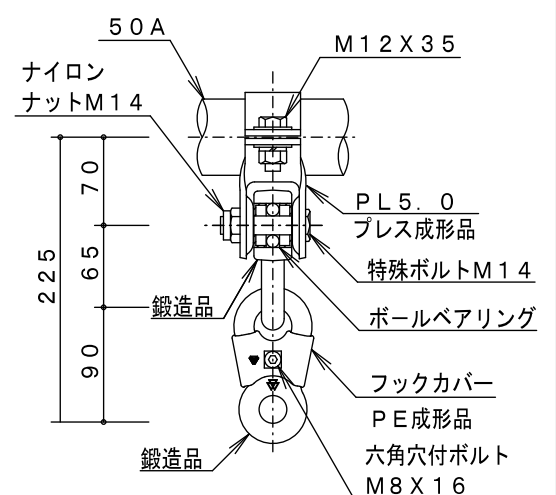
E詳細図 S=1/6
