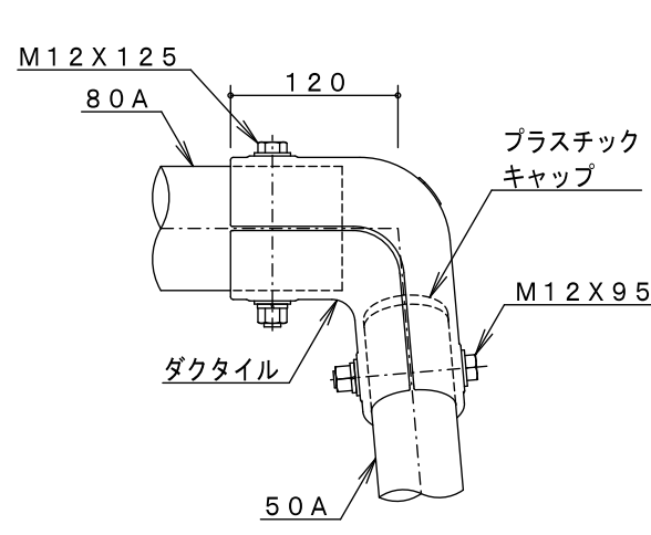
A詳細図 S=1/6
