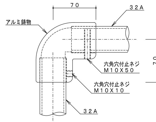
A詳細図 S = 1 / 3
