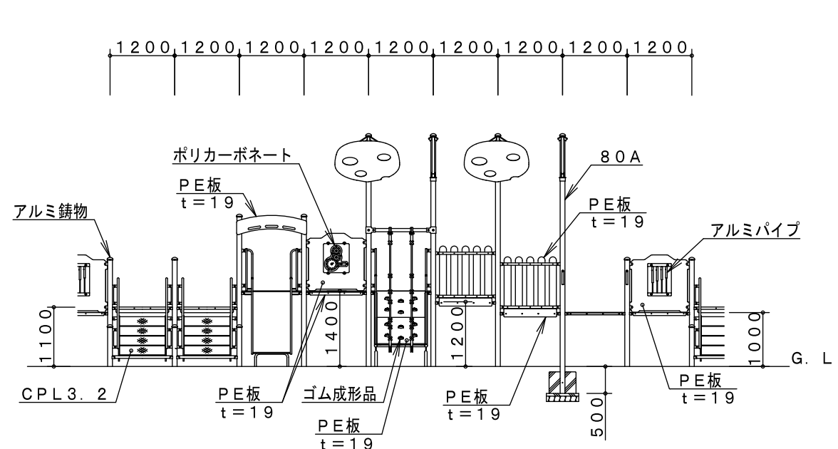
A-A' 展開図
