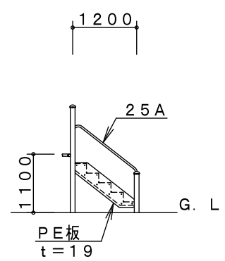
G 矢視図
