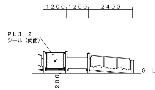
D-D' 展開図
