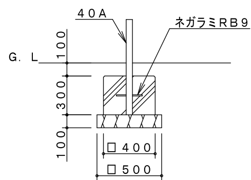
B基礎詳細図
