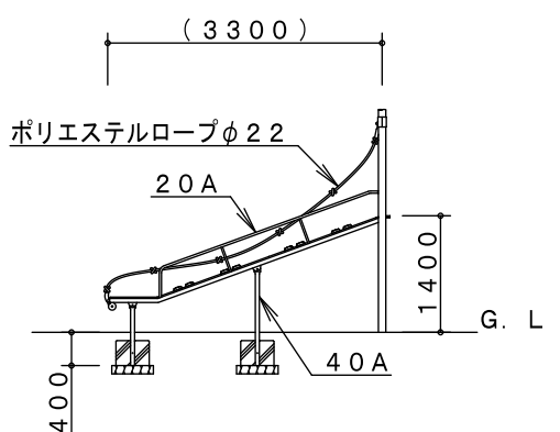
F 矢視図
