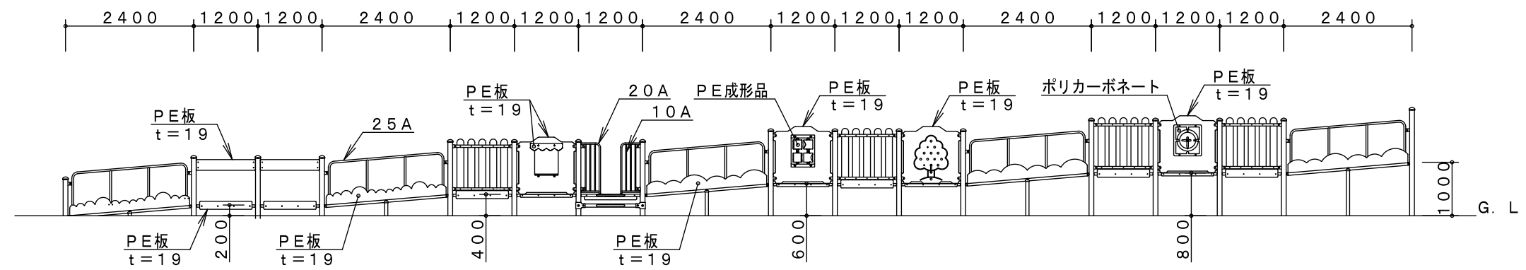
C-C' 展開図
