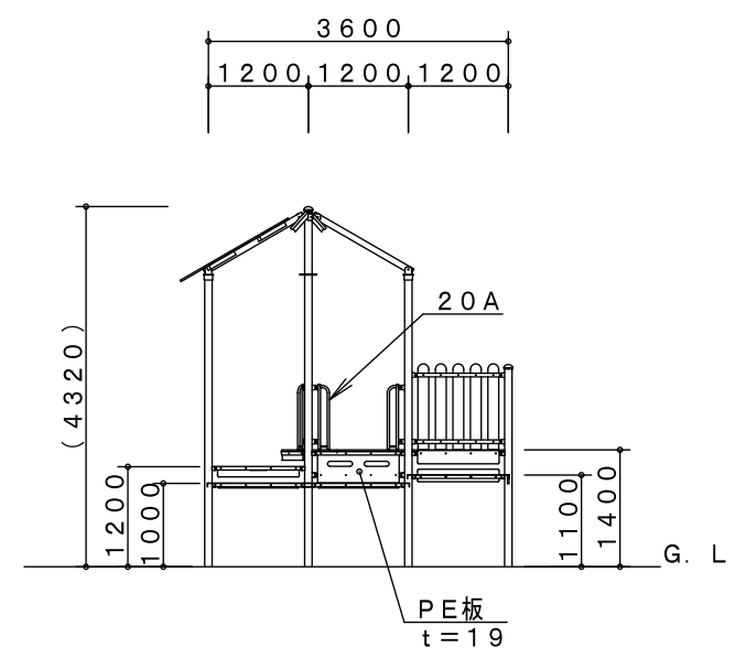
B-B' 矢視図
