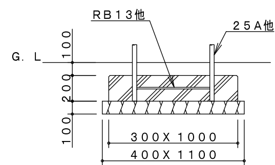
C基礎詳細図
