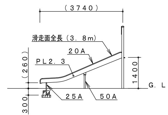
E 矢視図
