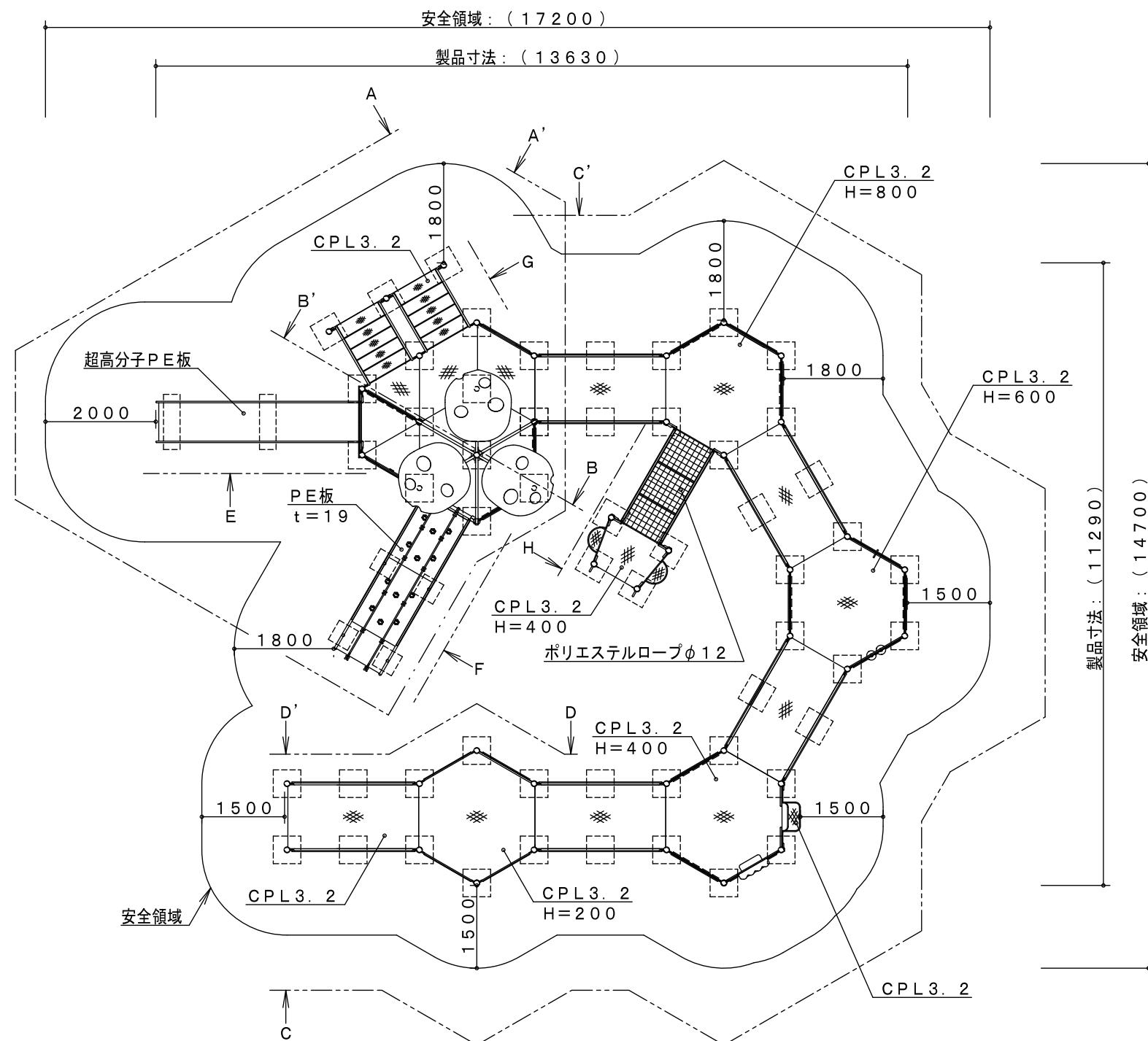
平面配置図・安全領域
