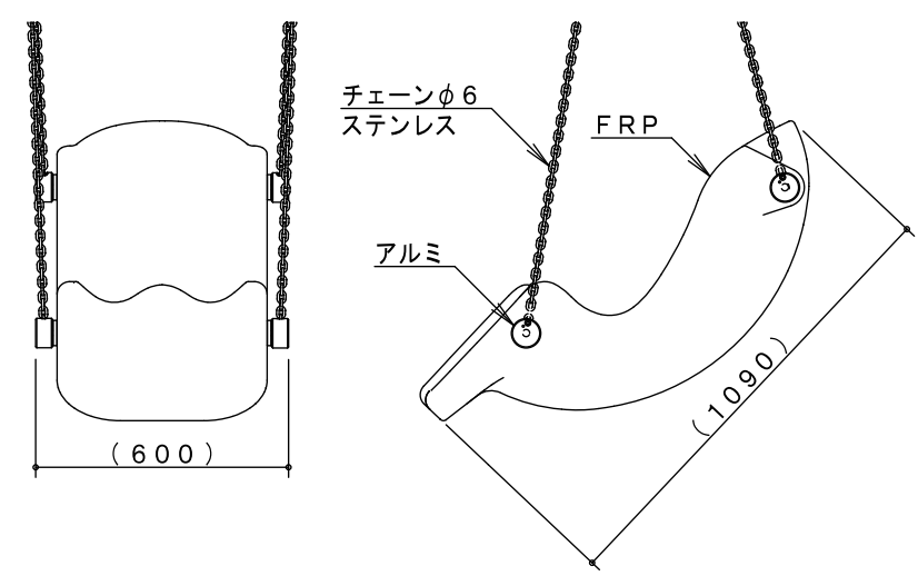
吊席 (A) 詳細図 S=1/20
