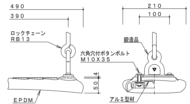
吊席 (B) 詳細図 S=1/6
