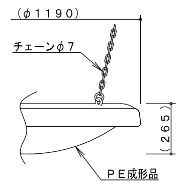
吊席 (C) 詳細図 S=1/20
