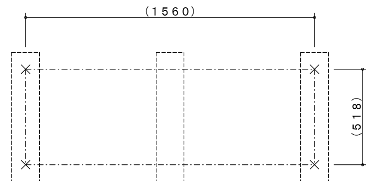
アンカー位置参考図 S = 1 / 20
