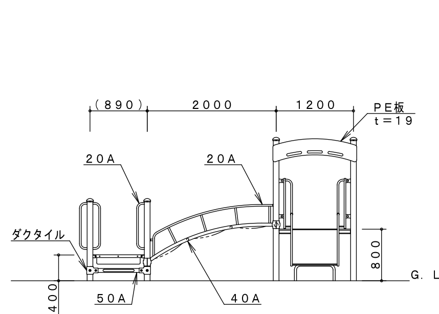
B-B' 矢視図
