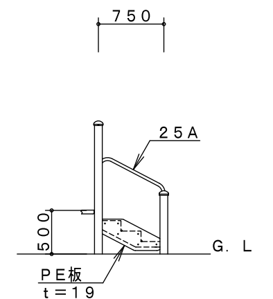
D-D' 矢視図
