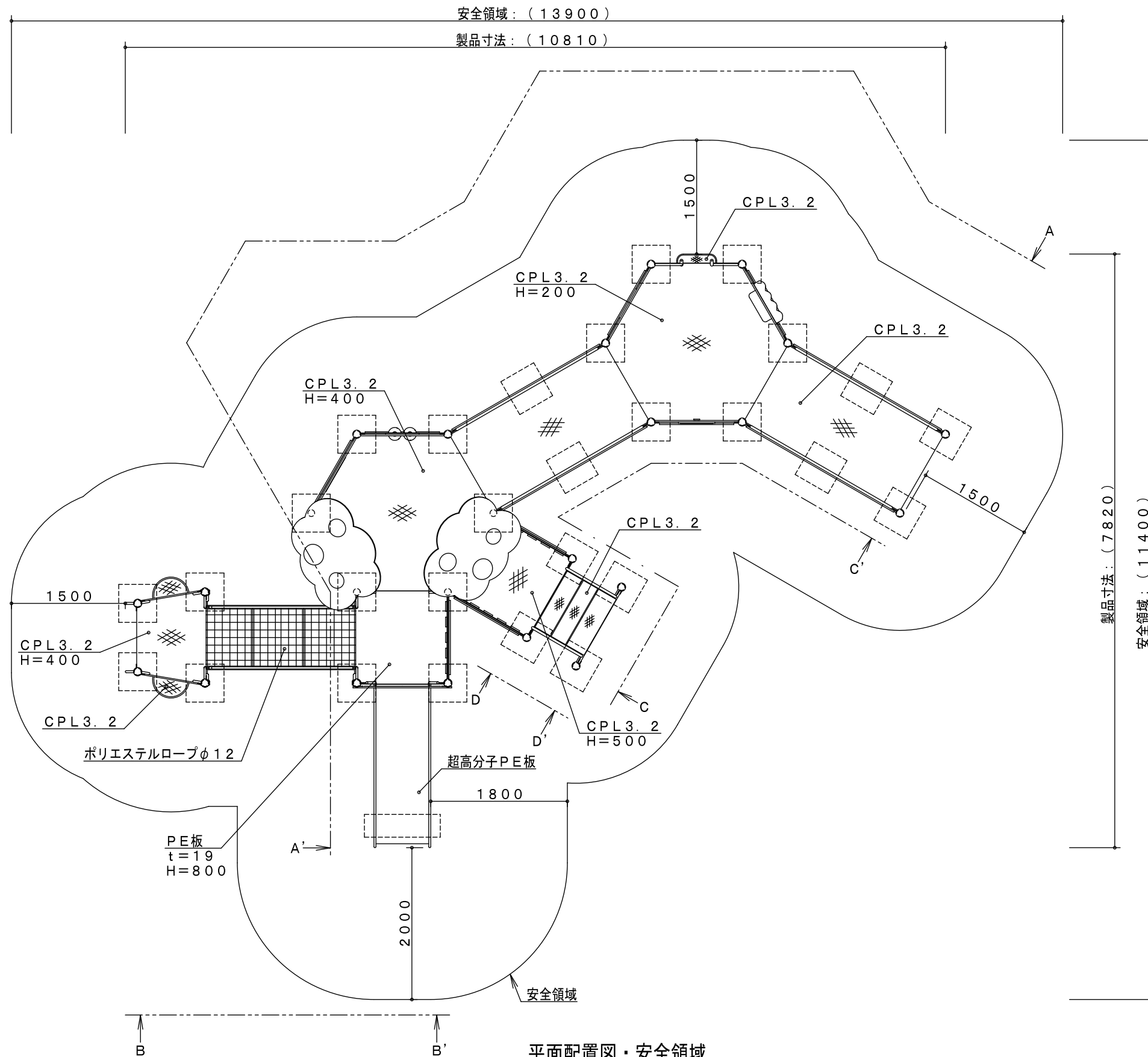
平面配置図・安全領域
