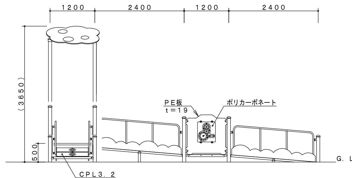
C-C' 展開図
