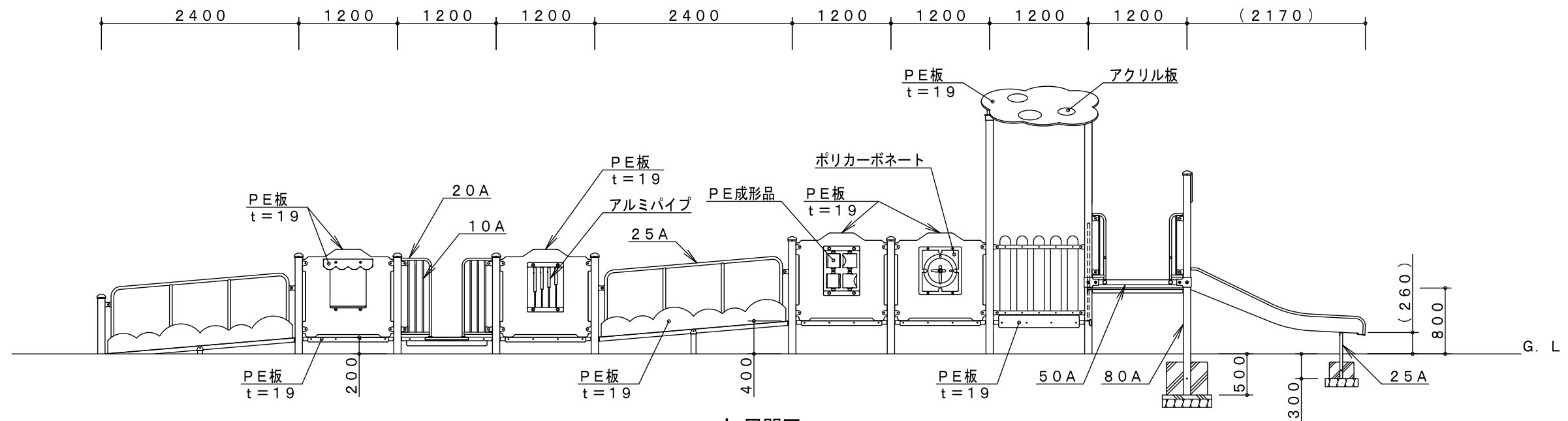
A-A' 展開図
