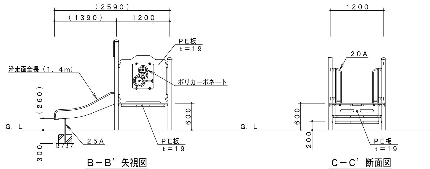
D-D' 展開図
