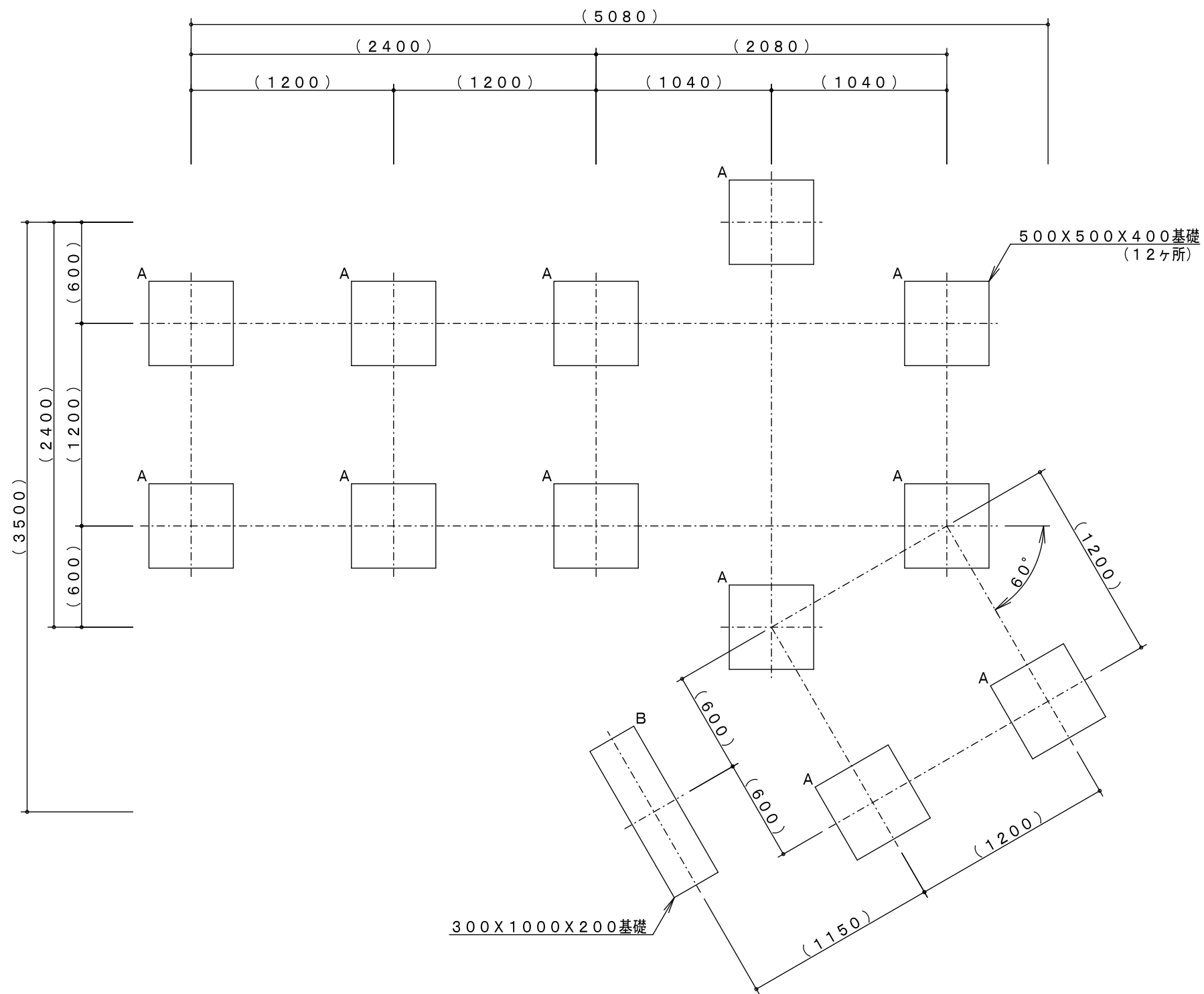
基礎平面図
