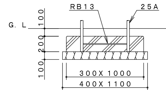
B基礎詳細図
