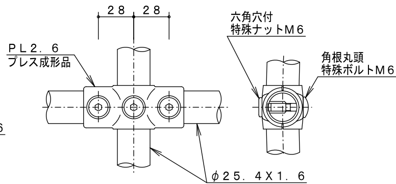
B 詳細図 S = 1 / 3
