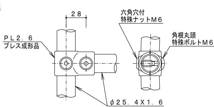
A 詳細図 S = 1 / 3
