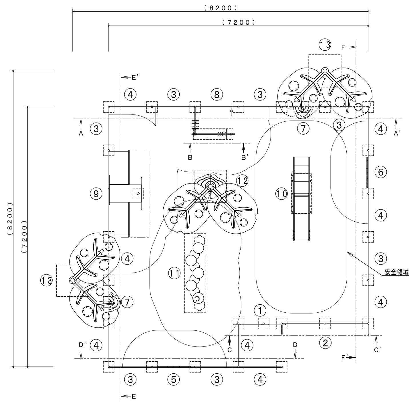
平面図
