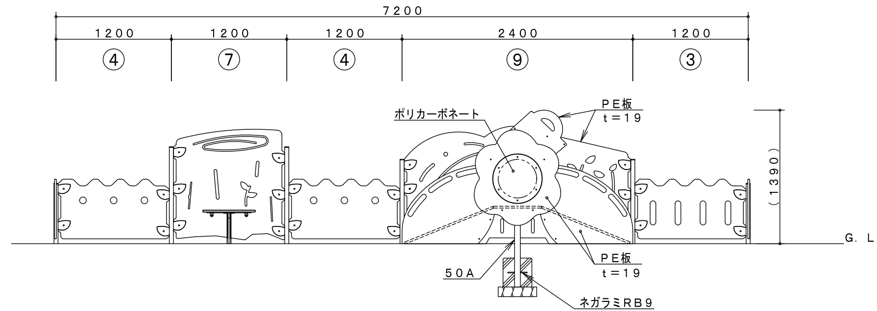
E-E' 矢視図
