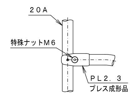
C詳細図 S=1/6
