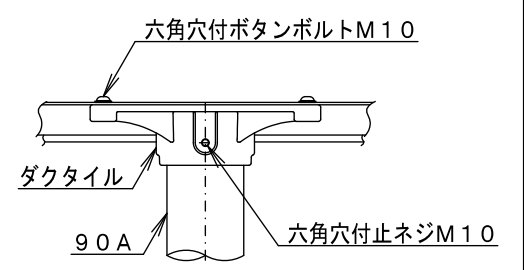
D詳細図 S=1/10
