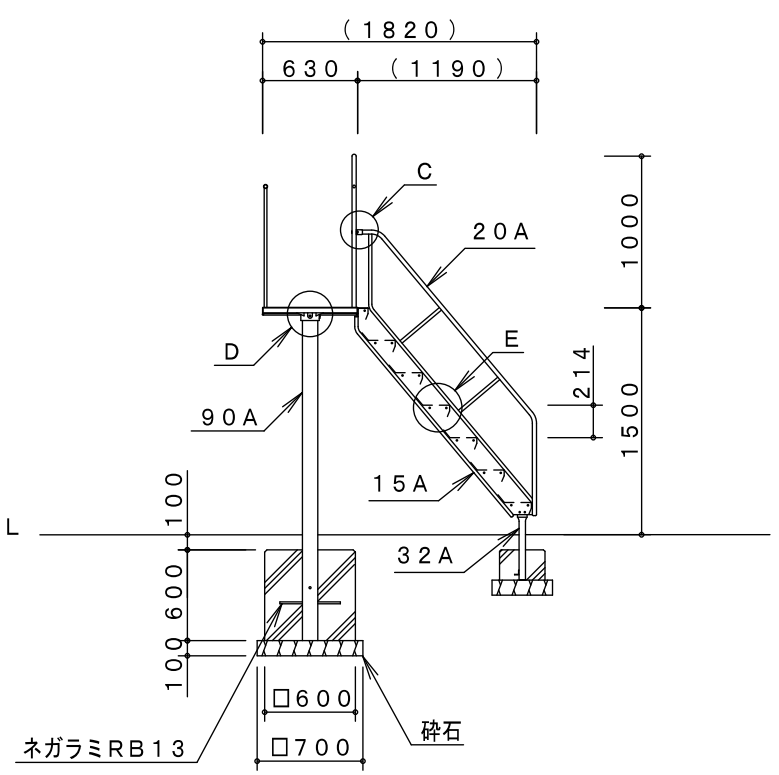
A矢視図
