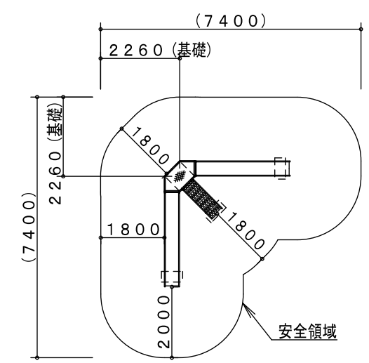
安全領域 S=1/150
