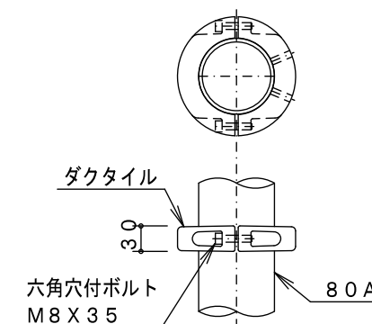
B詳細図 S=1/8
