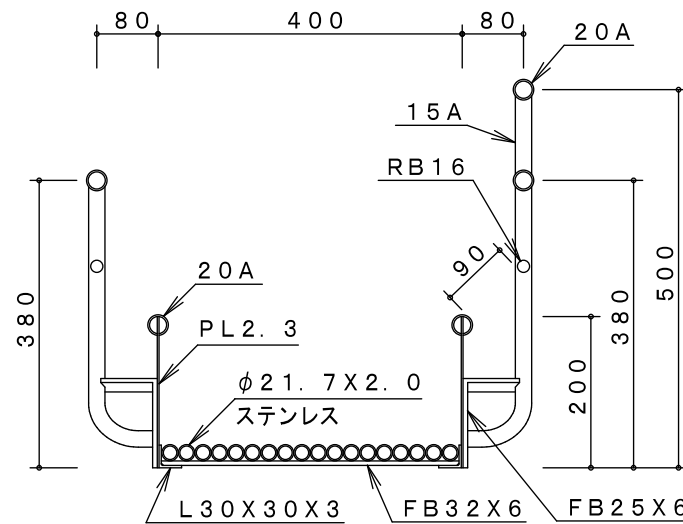
滑面上部断面図 S=1/10
