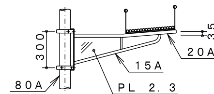
第2・8段 詳細図 S=1/30
