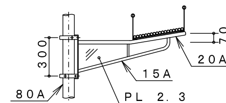
第3～7段 詳細図 S=1/30
