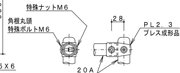
A詳細図 S=1/5
