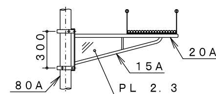
第1段 詳細図 S=1/30
