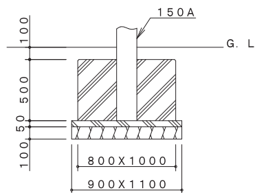
B基礎詳細図 S=1/30
