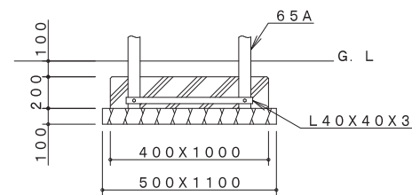
C基礎詳細図 S=1/30
