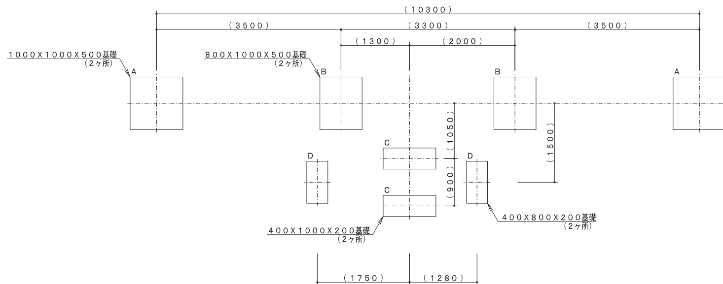
基礎平面図
