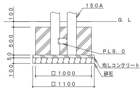
A基礎詳細図 S=1/30
