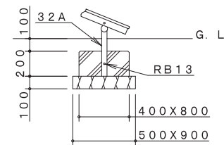
D基礎詳細図 S=1/30
