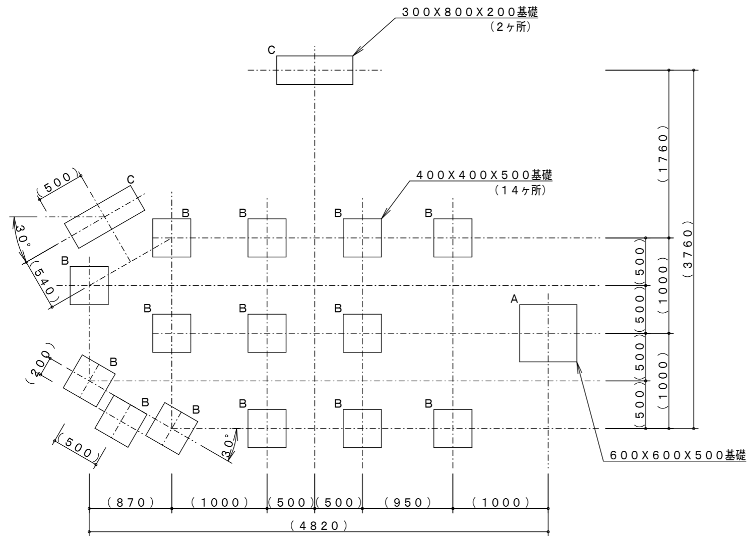
基礎平面図
