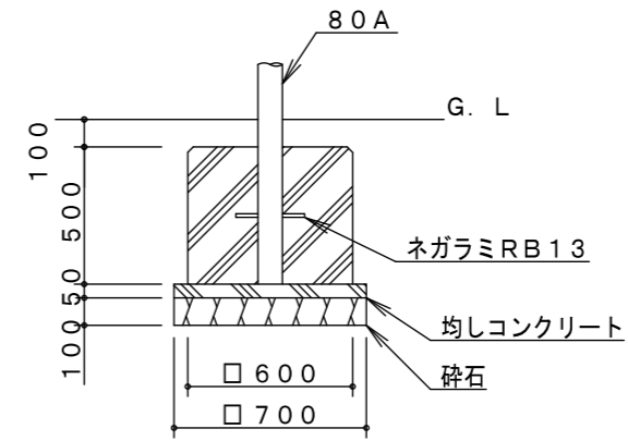
A基礎詳細図 S=1/30
