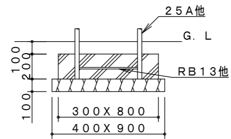
C基礎詳細図 S=1/30
