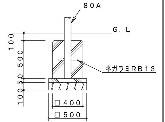
B基礎詳細図 S=1/30
