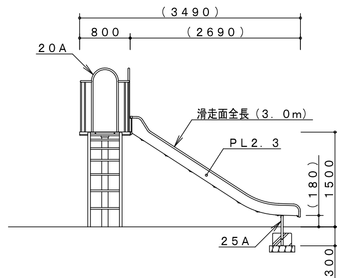
C-C' 矢視図
