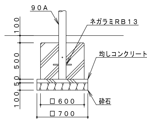
A基礎詳細図
