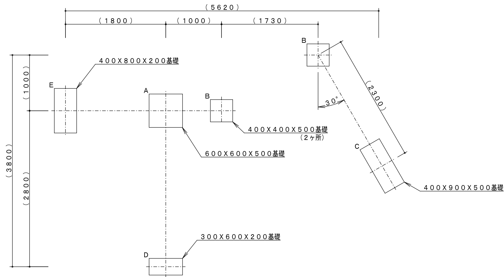
基礎平面図 S=1/40
