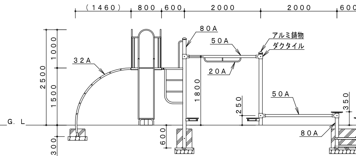
A-A' 展開図
