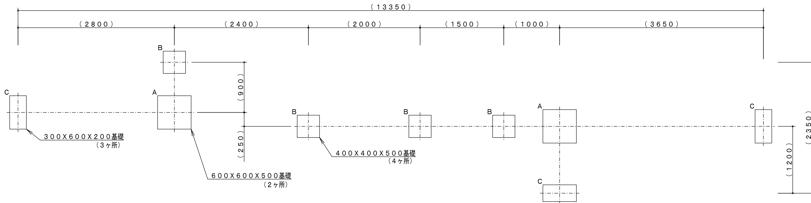
基礎平面図 S = 1 / 4 0
