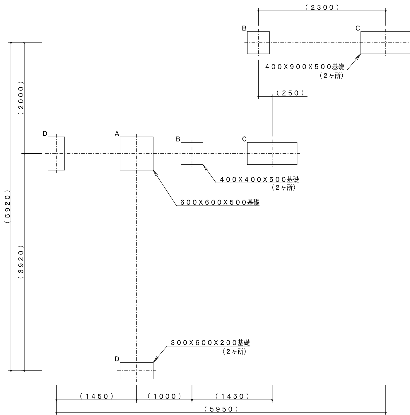
基礎平面図 S = 1 / 40
