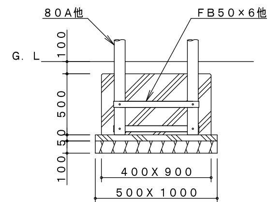
C基礎詳細図
