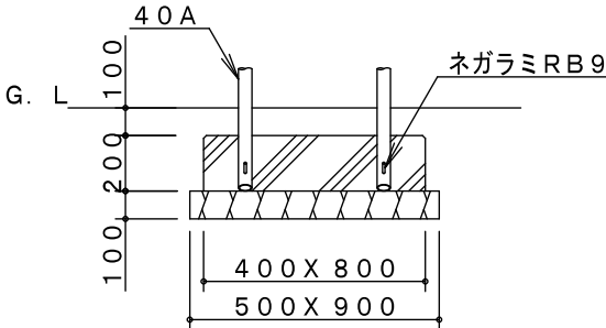
D基礎詳細図
