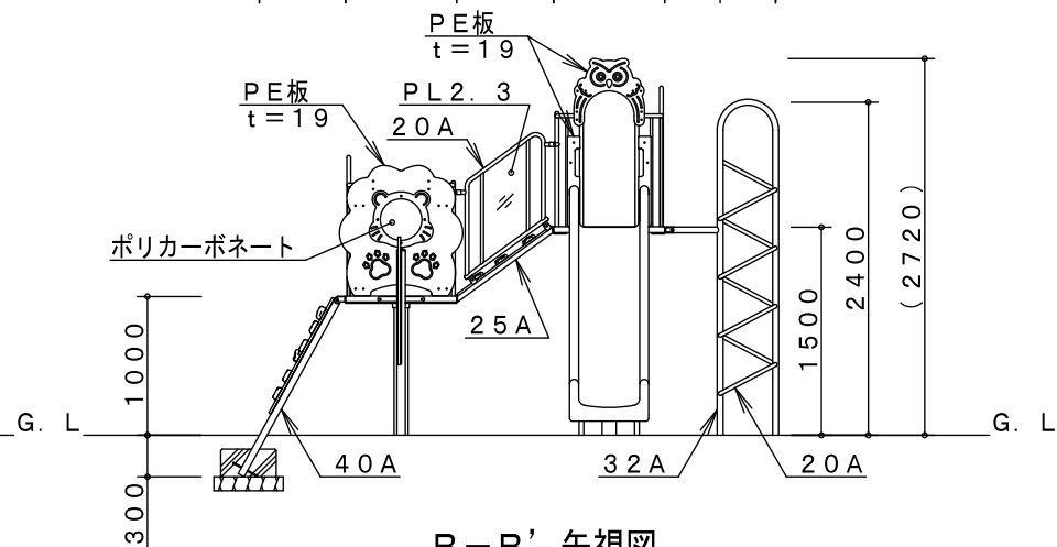
B-B' 矢視図
