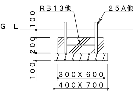
C基礎詳細図
