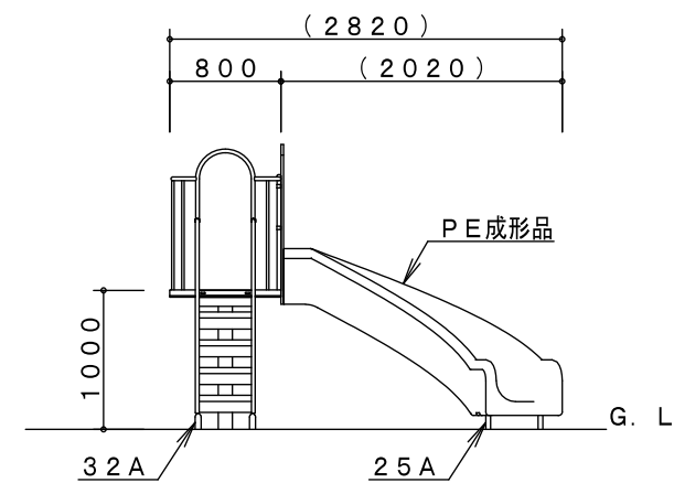
A-A' 矢視図
