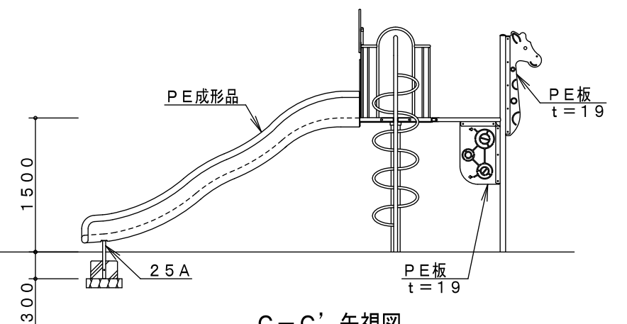
C-C' 矢視図
