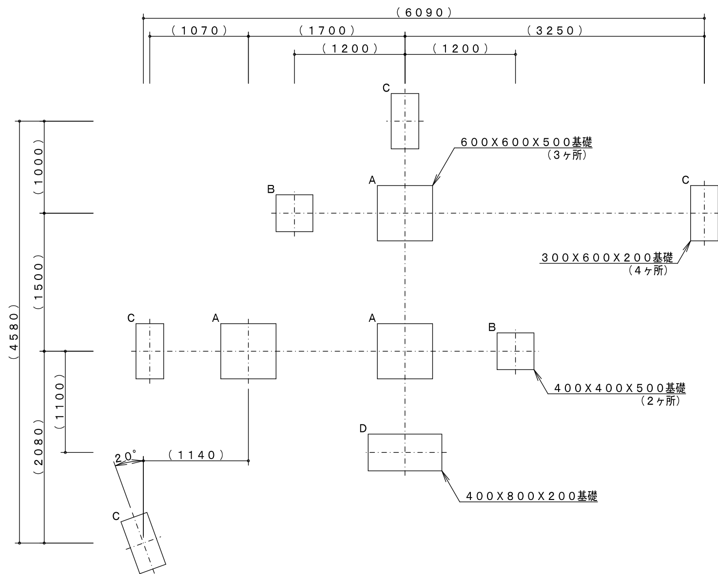
基礎平面図 S = 1 / 40
