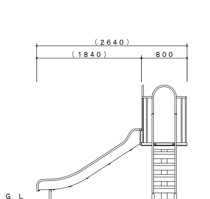
A-A' 矢視図
