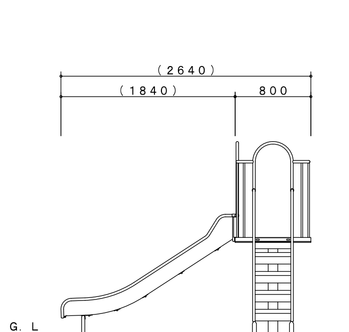
A-A' 矢視図
