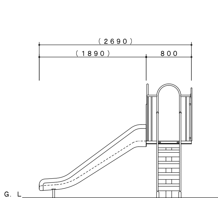
A-A' 矢視図
