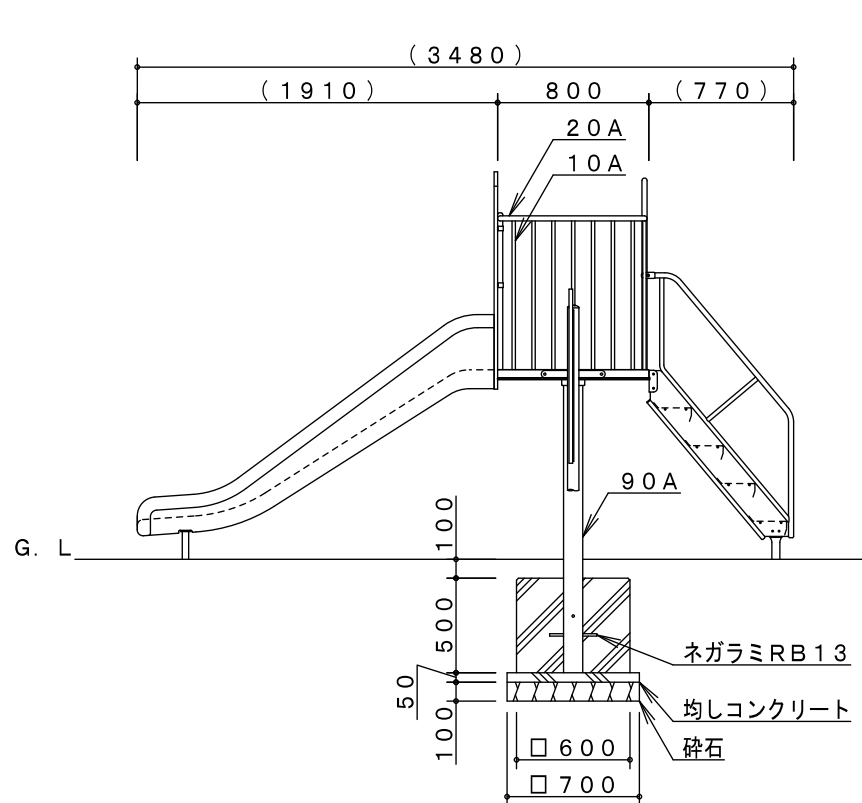
A-A' 矢視図
