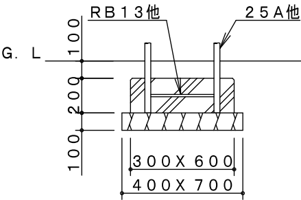
B 基礎詳細図
