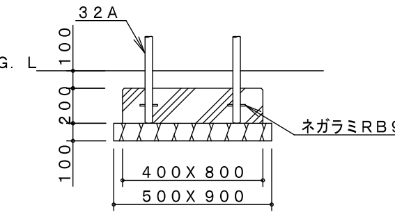
C 基礎詳細図
