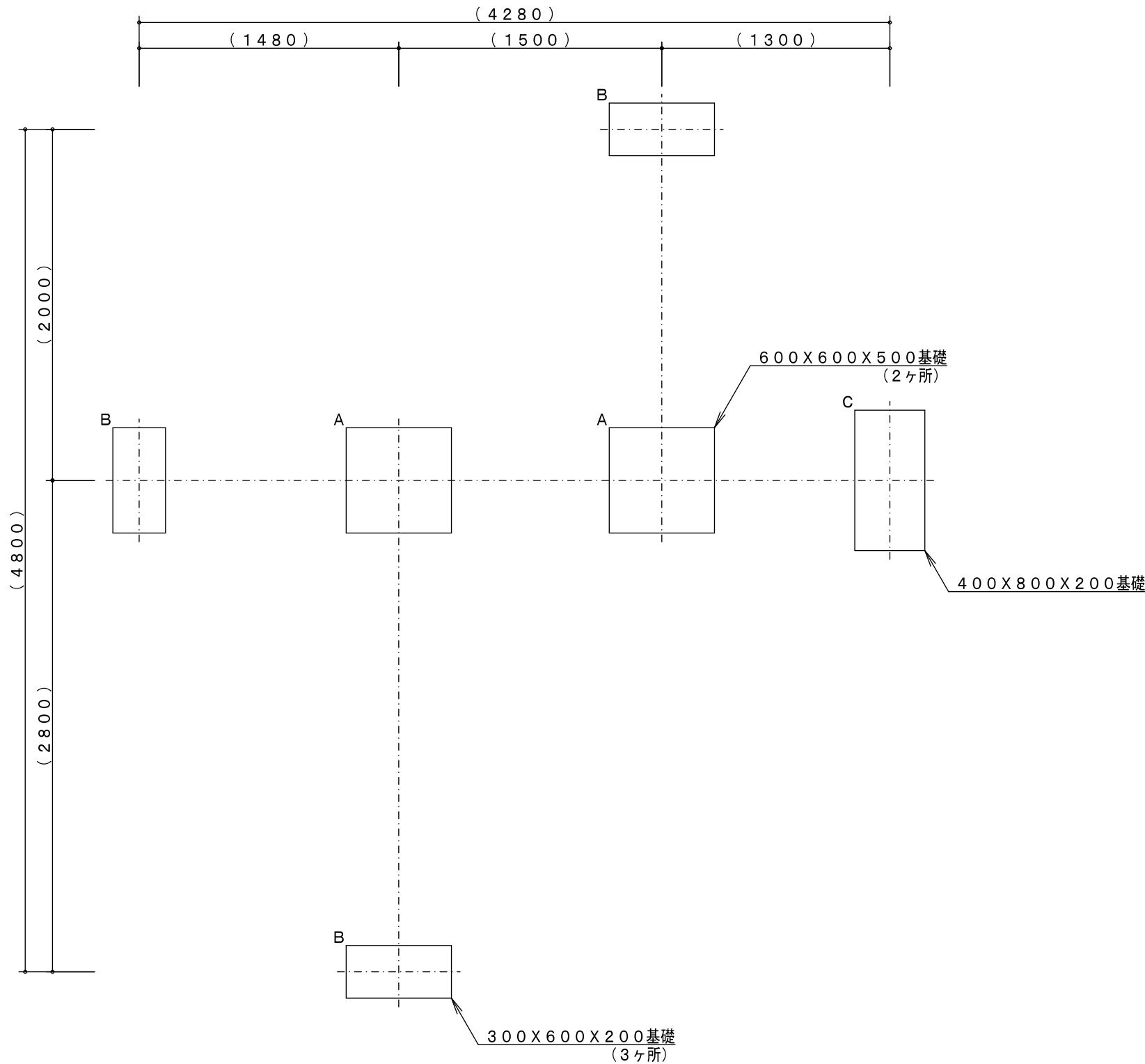
基礎平面図
