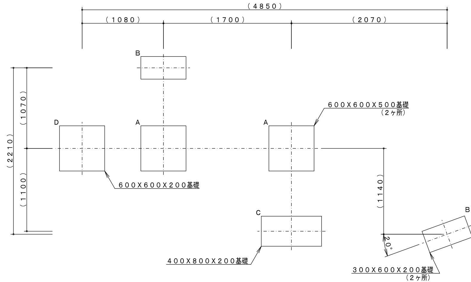
基礎平面図
