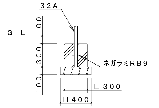
F基礎詳細図
