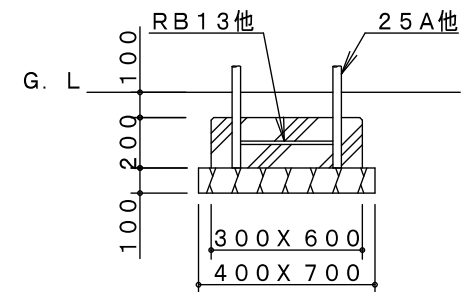
B基礎詳細図
