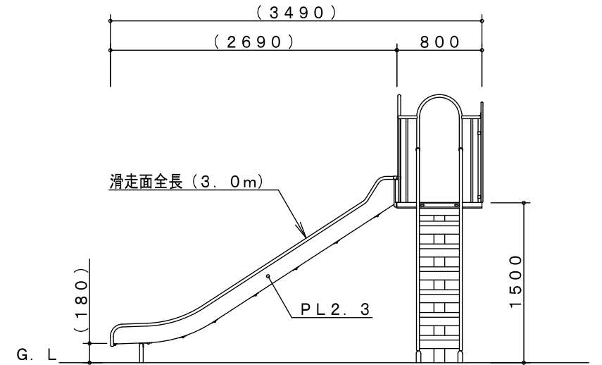
A-A' 矢視図
