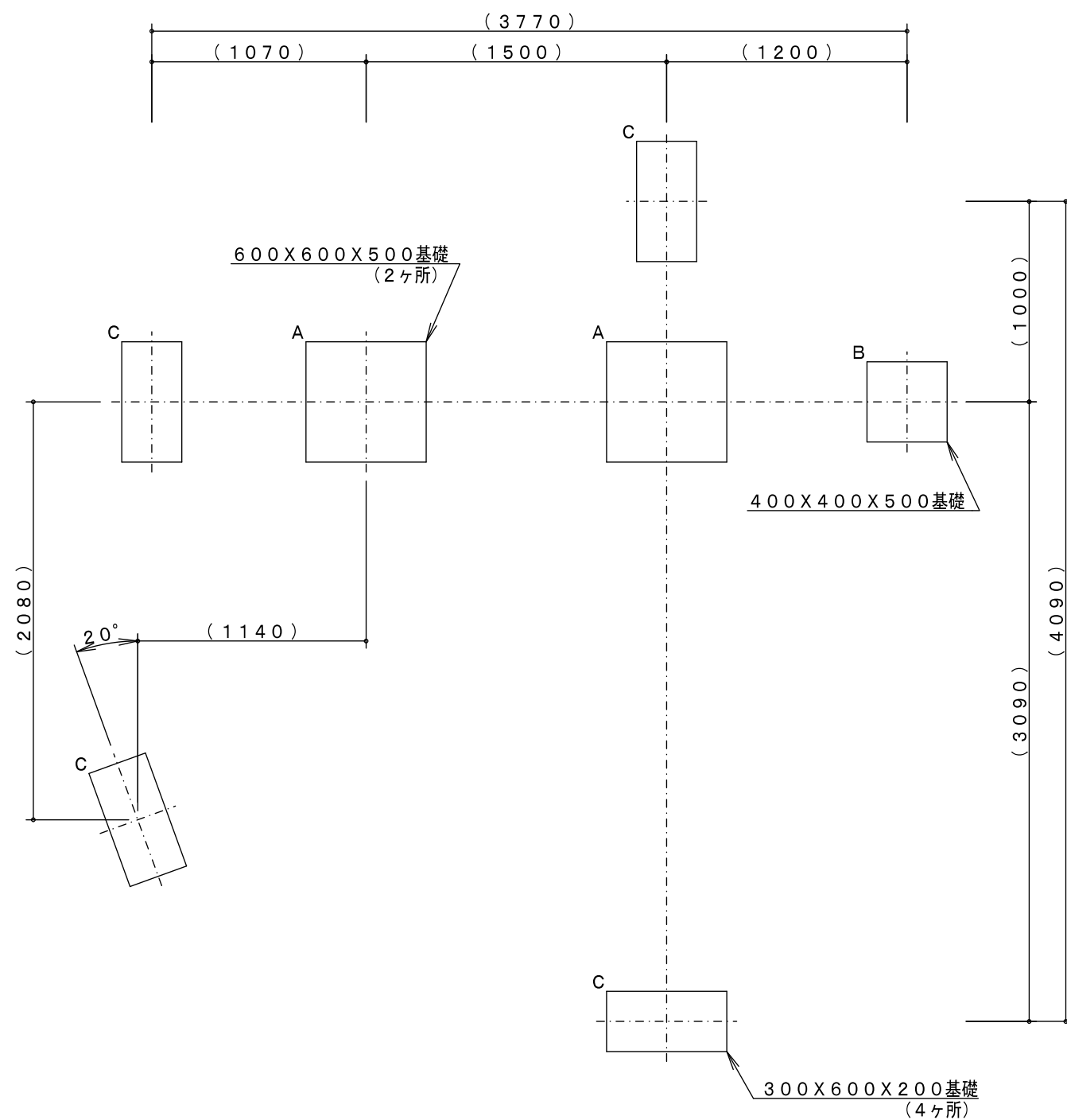
基礎平面図
