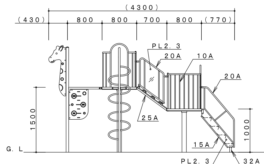
A-A' 矢視図
