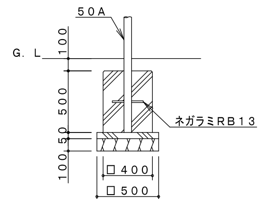
B基礎詳細図
