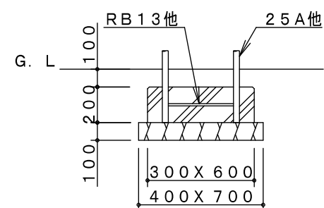
C基礎詳細図
