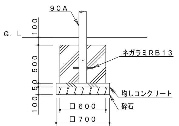
A基礎詳細図
