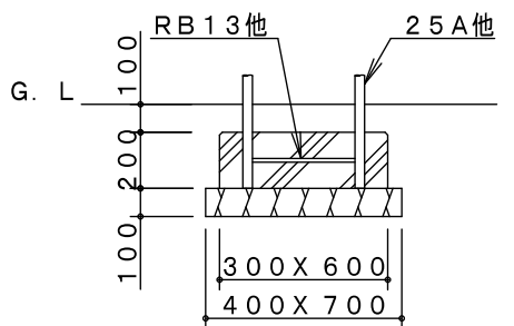
B基礎詳細図
