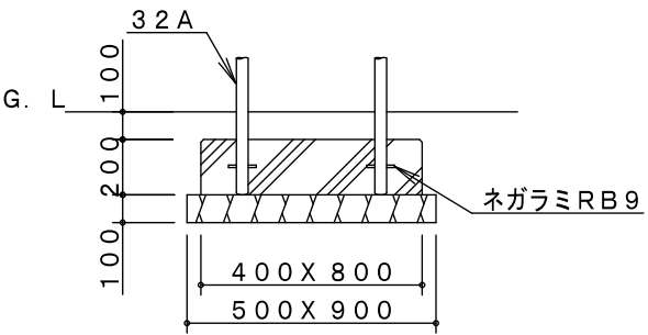
C基礎詳細図
