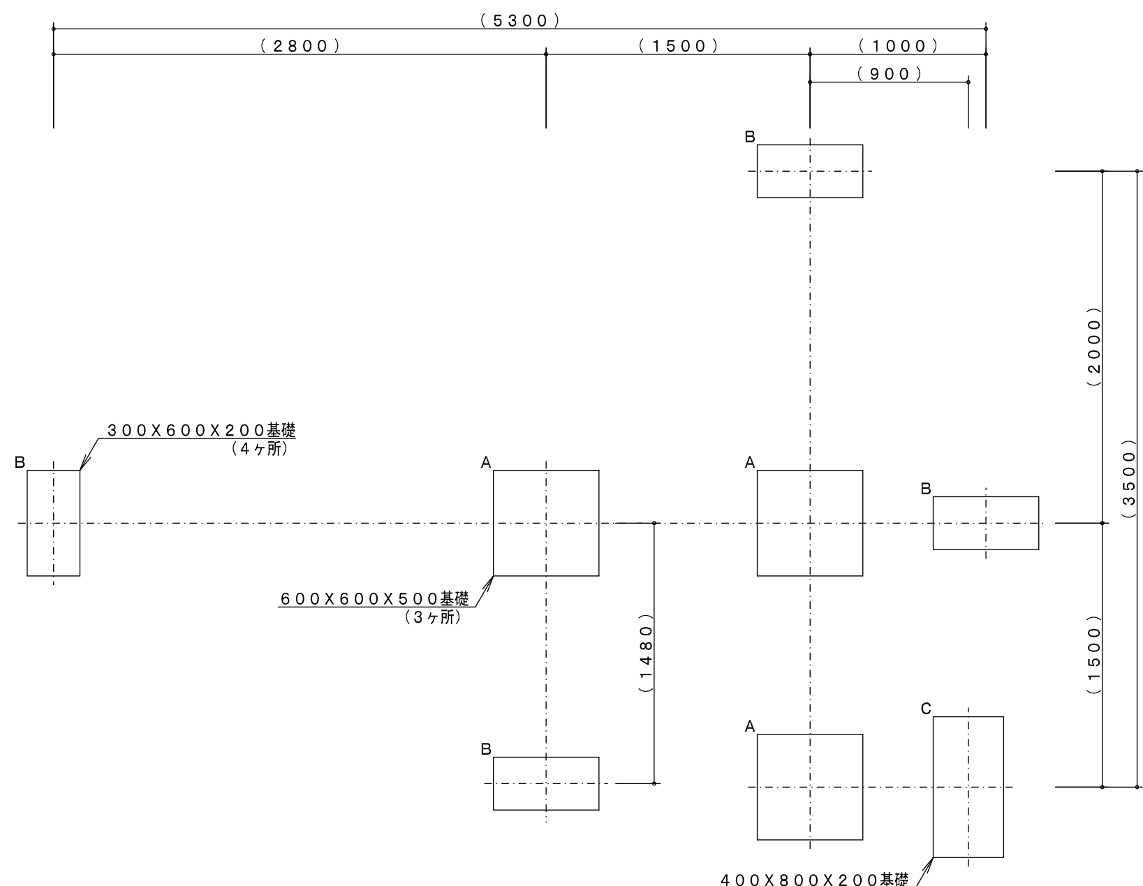
基礎平面図
