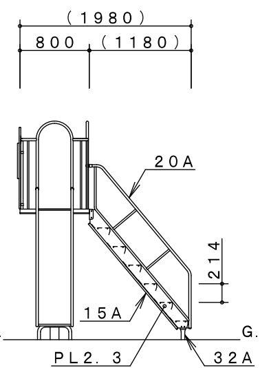
C-C' 矢視図
