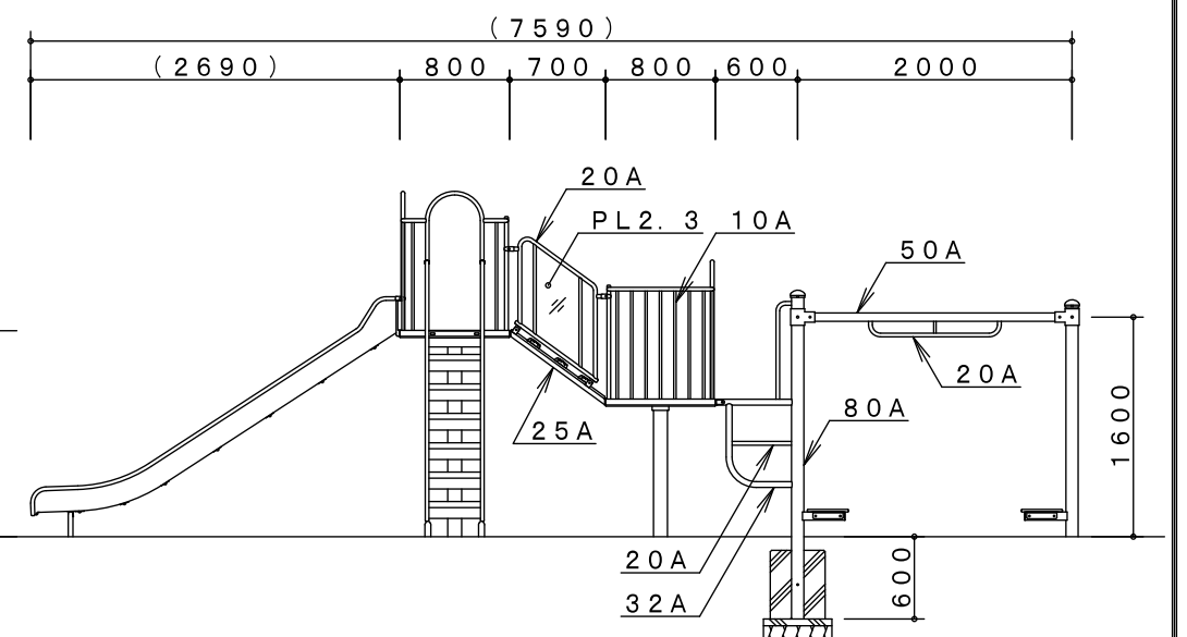
D-D' 矢視図
