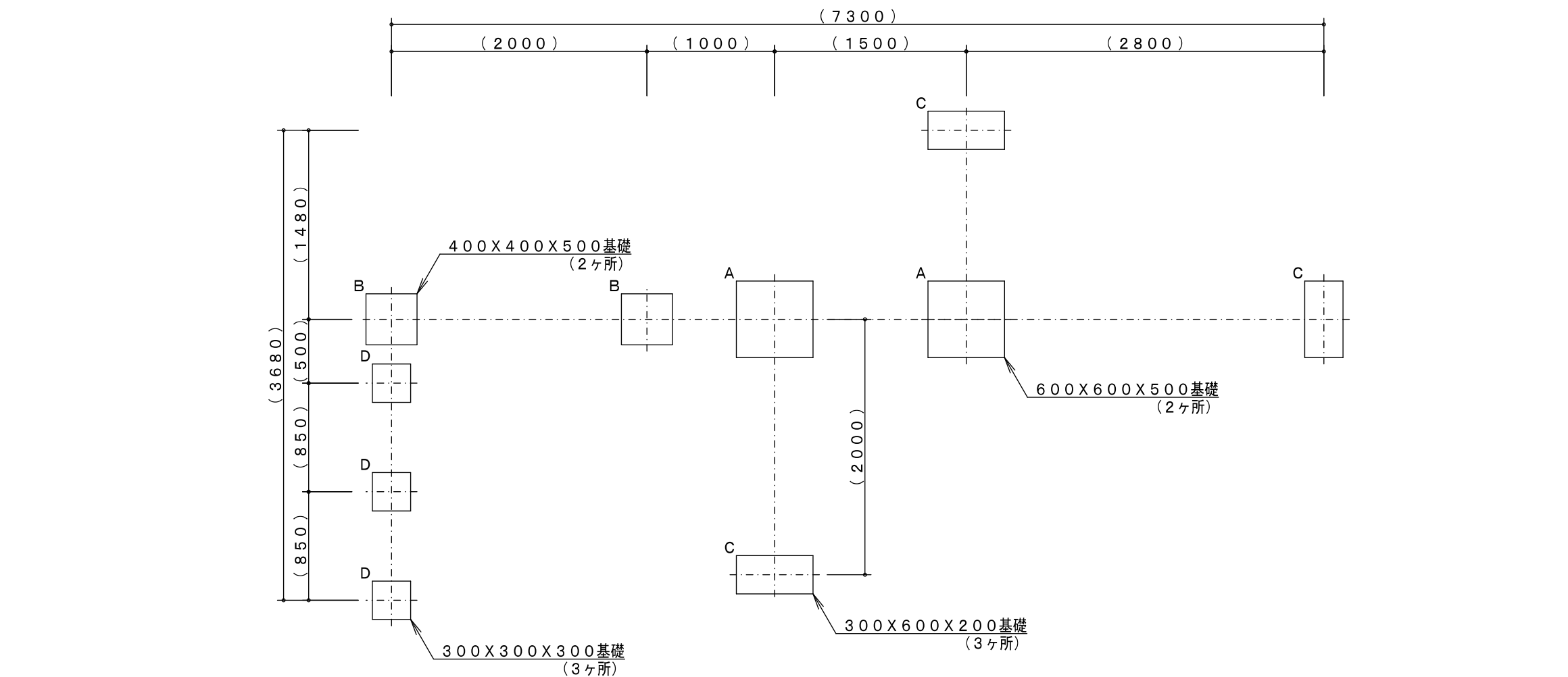
基礎平面図 S = 1 / 4 0
