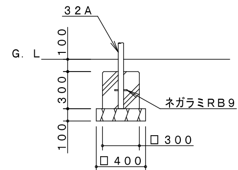
D基礎詳細図
