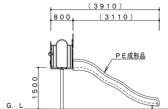
A-A' 矢視図
