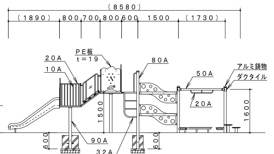
C-C' 矢視図
