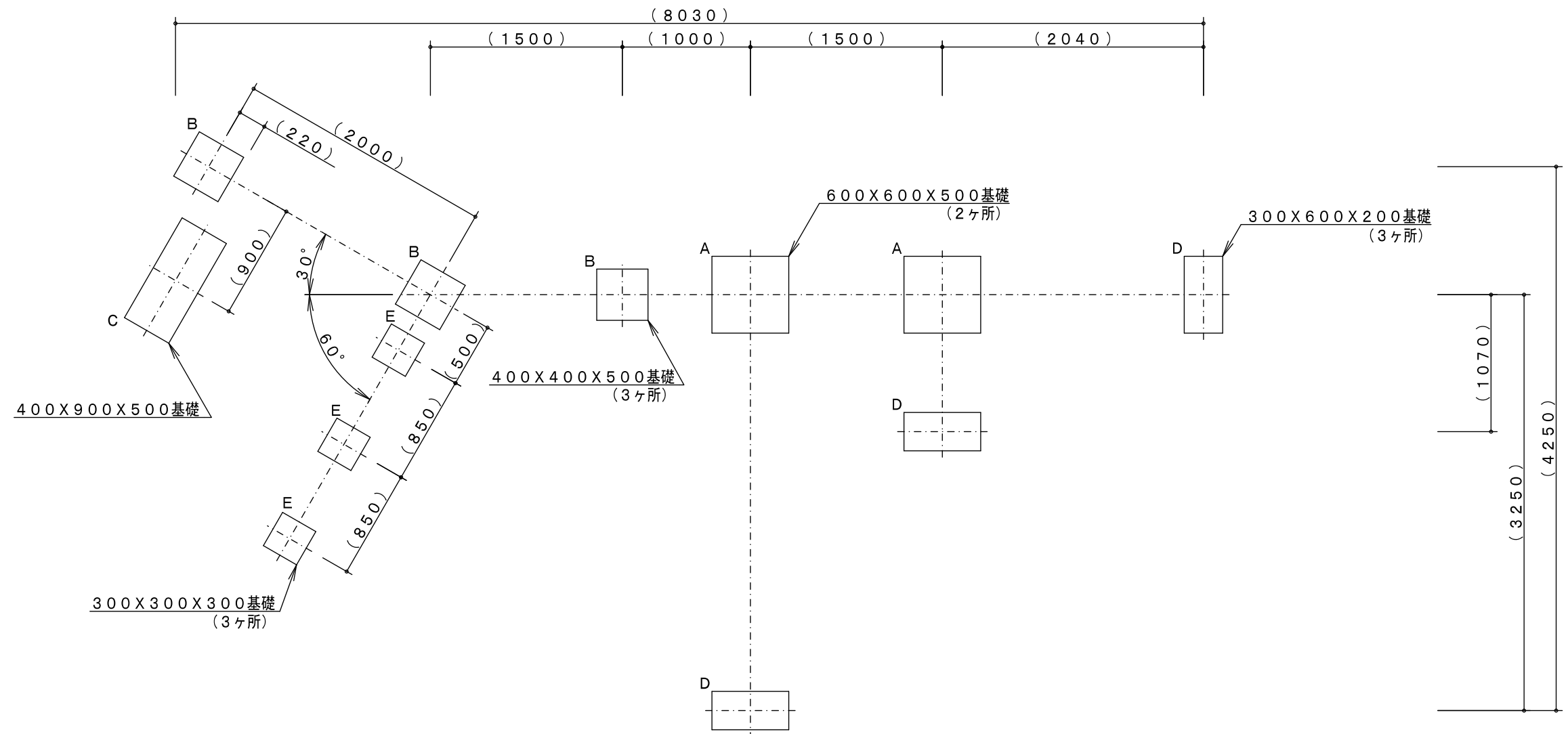
基礎平面図 S = 1 / 4 0
