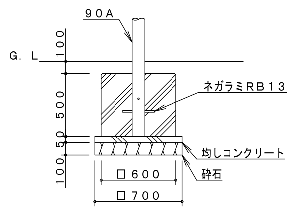
A基礎詳細図
