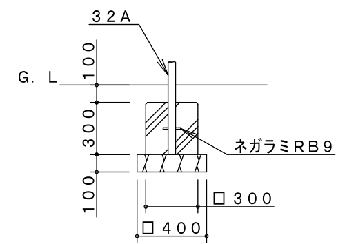
E基礎詳細図
