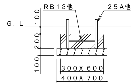
C基礎詳細図
