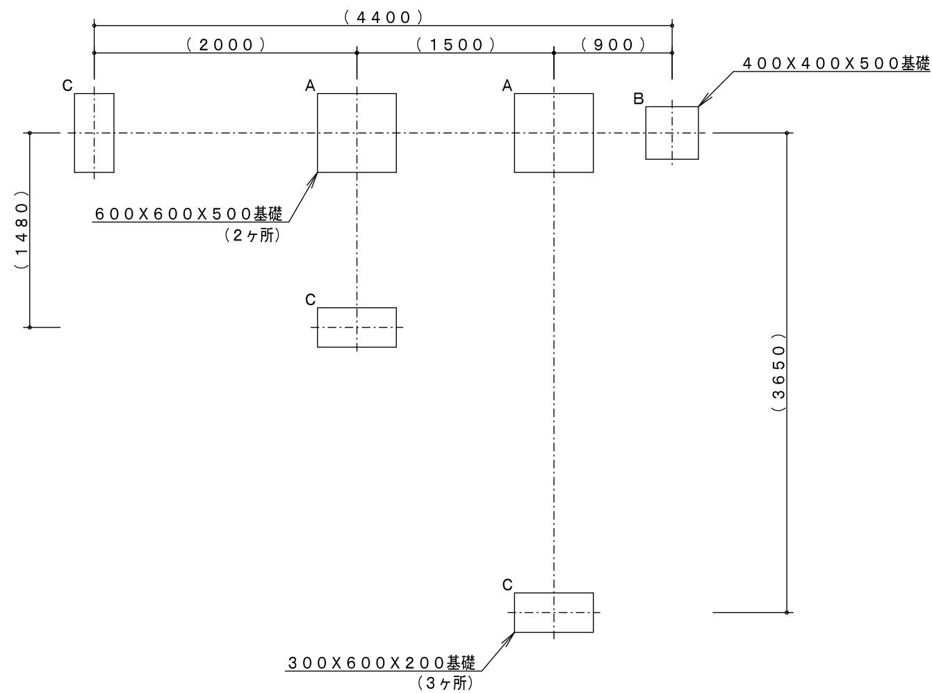
基礎平面図 S=1/40
