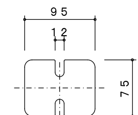
A詳細図 S=1/5
